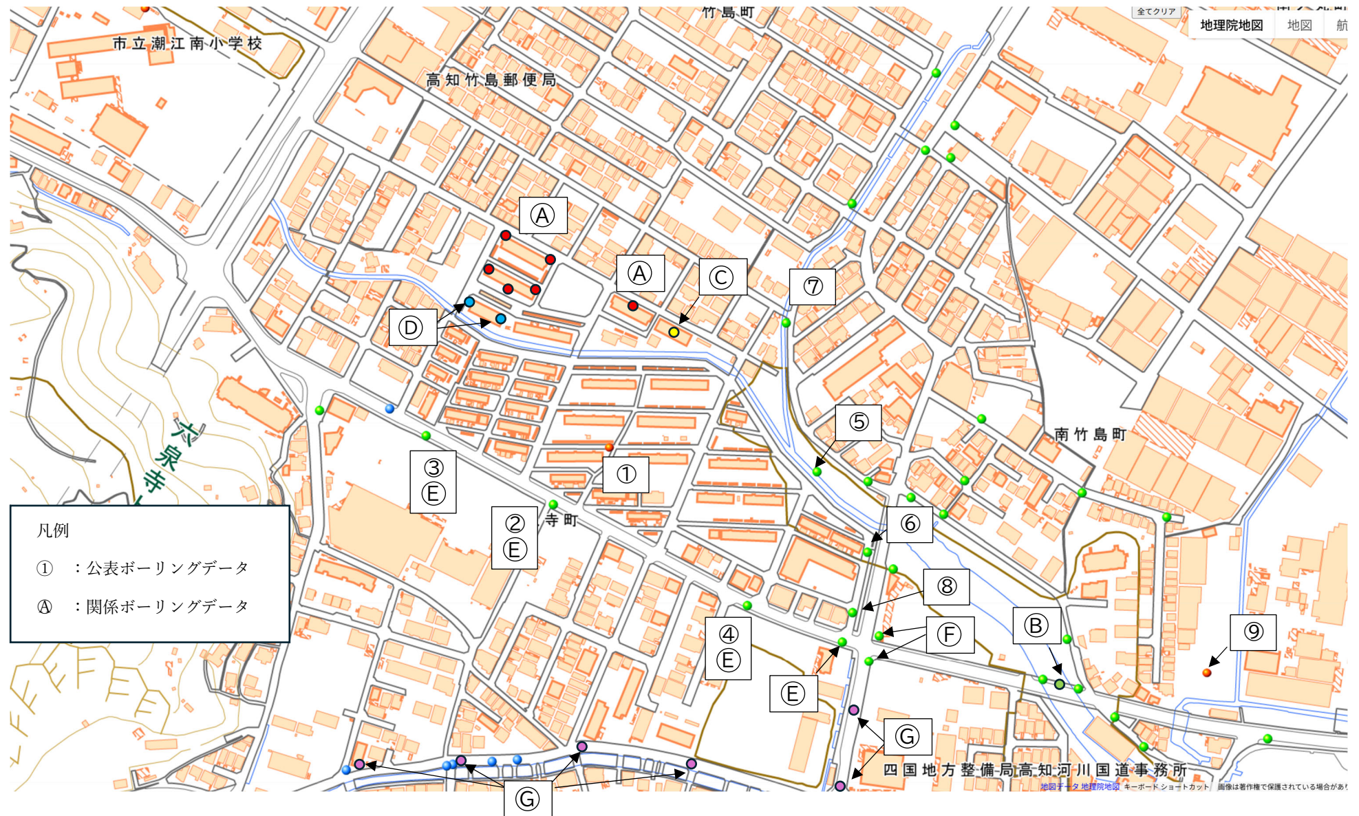
別紙 6 - 1 : 地質調査結果 (事業用地及び周辺 公表ボーリングデータ・関係ボーリングデータ位置図)
