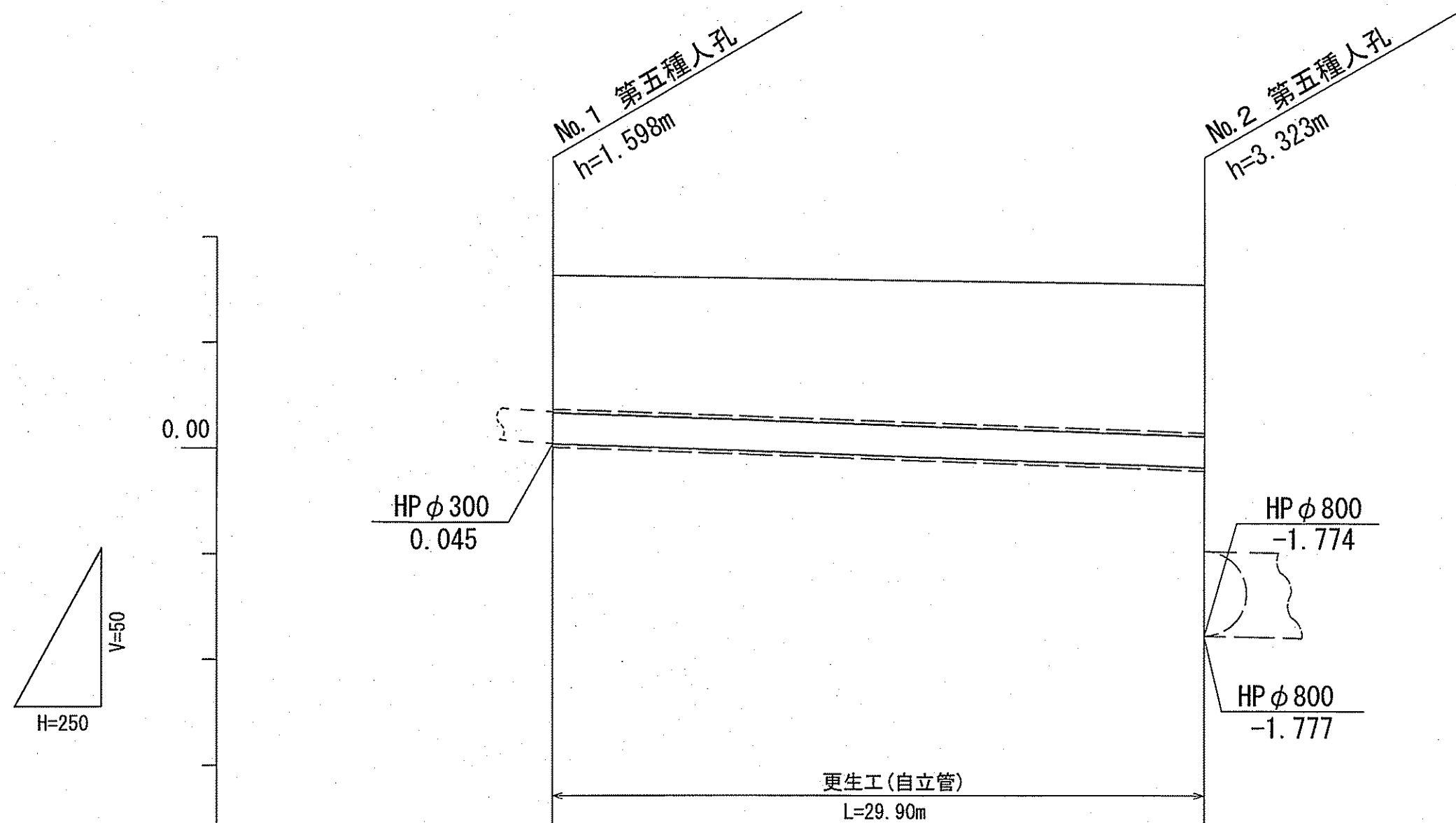
縦断図 V=1:50 H=1:250
