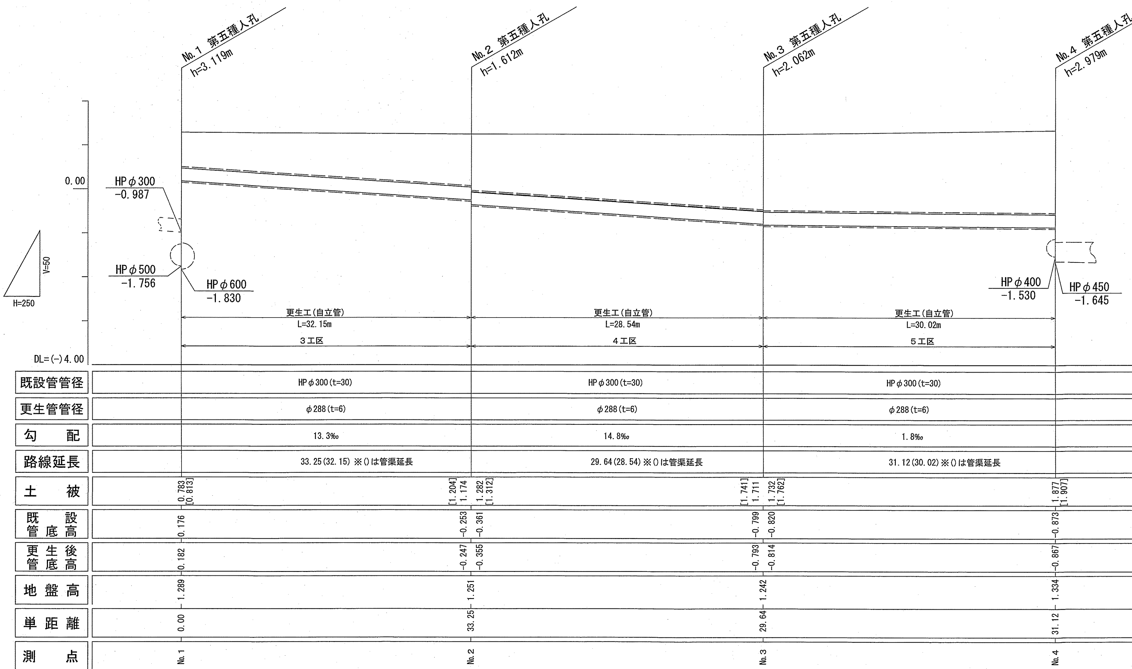
縦断図 V=1:50 H=1:250
