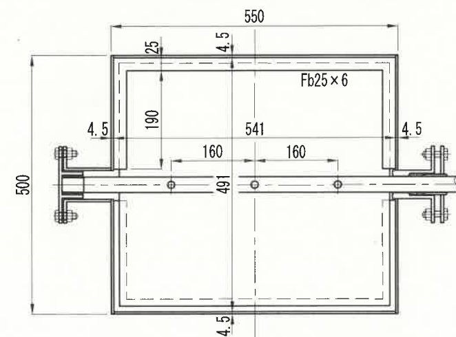
A断面
