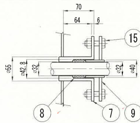
D詳細 (S=1:5)
