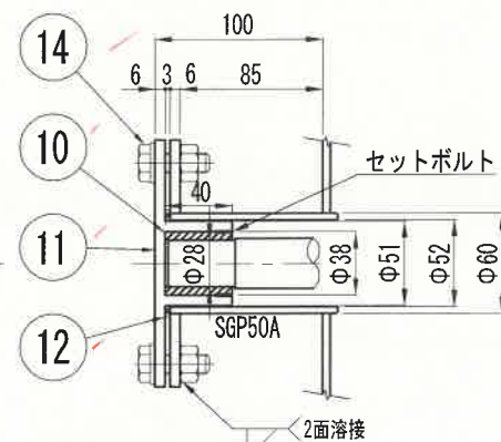
C詳細 (S=1:5)
