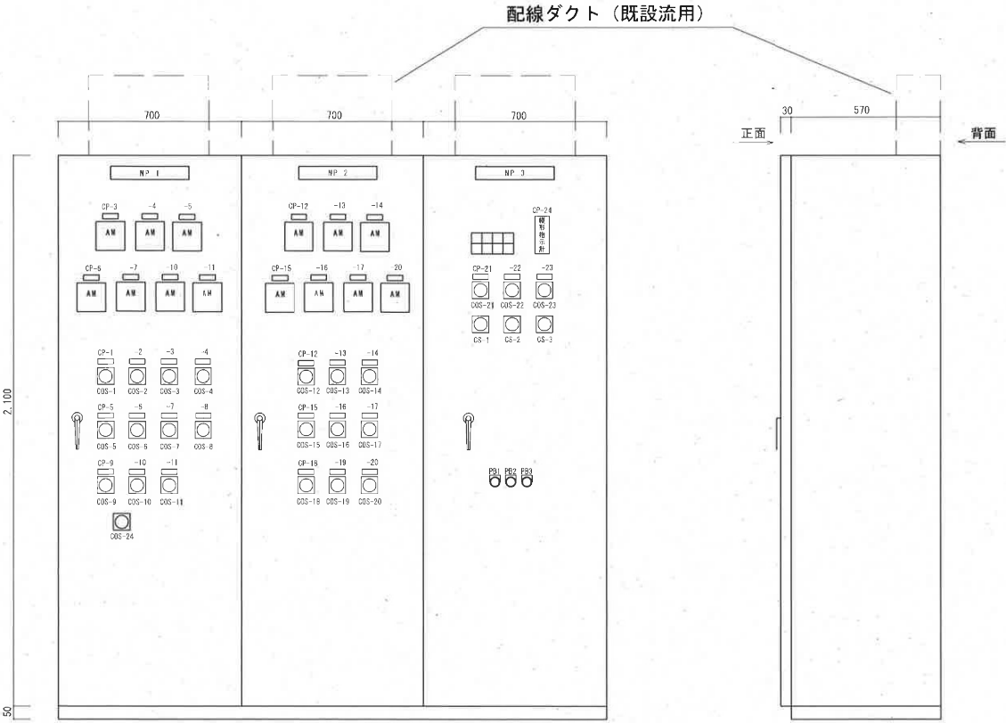
正面図
