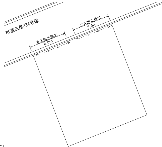
平面図(既存施設撤去) Scale 1:200
