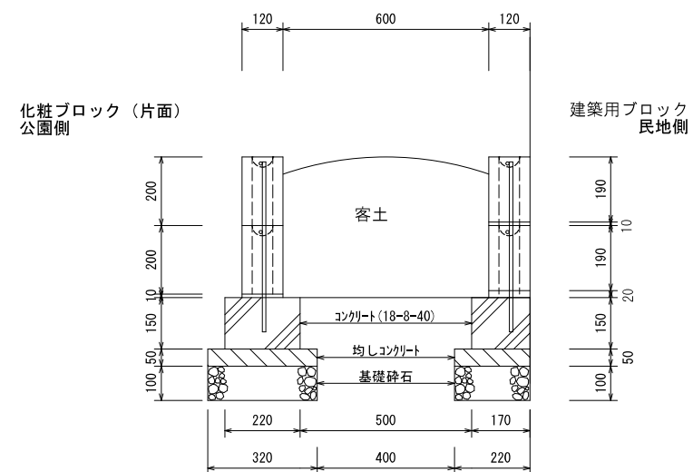
構造図 (花壇) Scale 1:20
