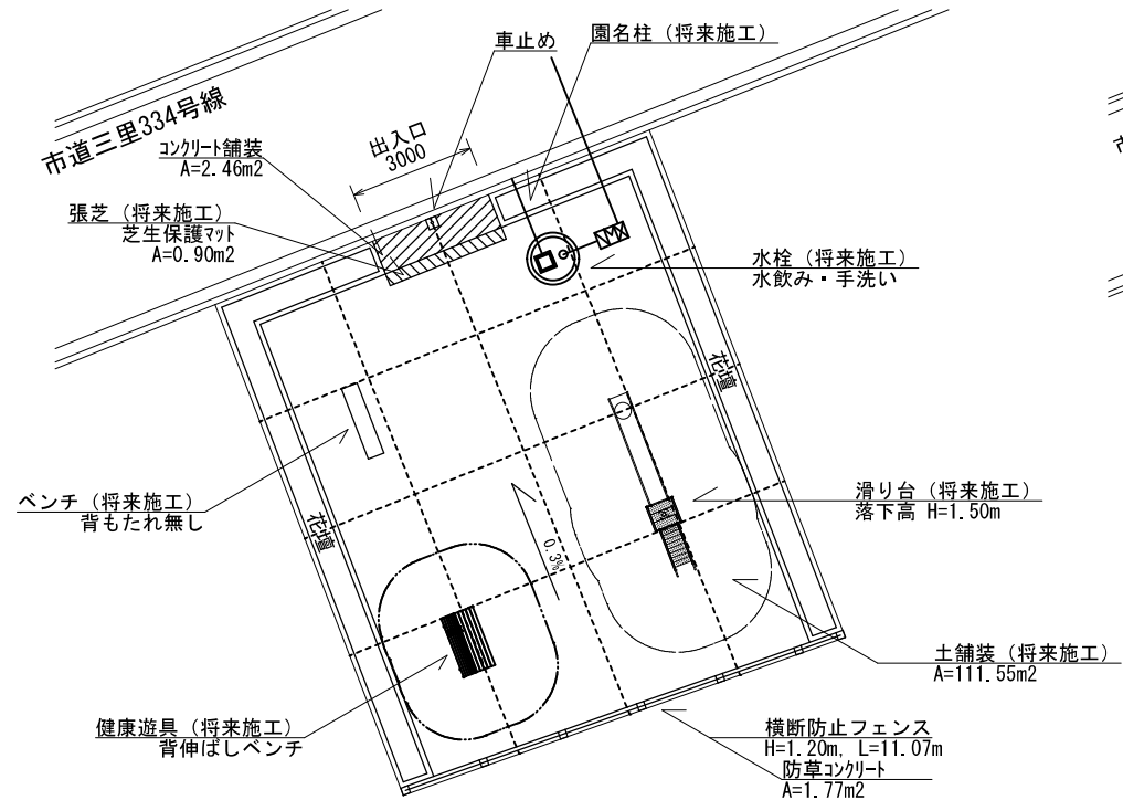
平面図(整備計画) Scale 1:200
