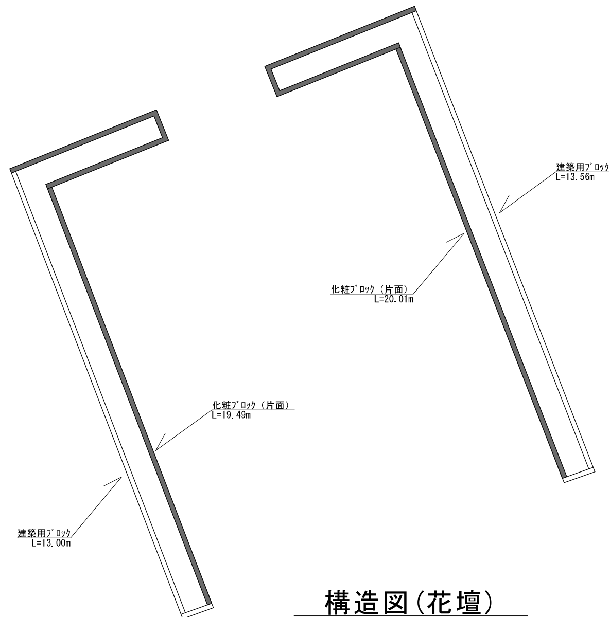
平面図(花壇) Scale 1:100
