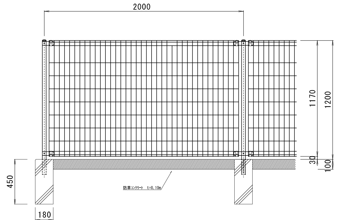
参考：構造図(フエンス) Scale 1:20
