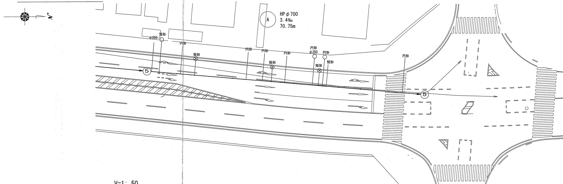
平面図 S=1:250
