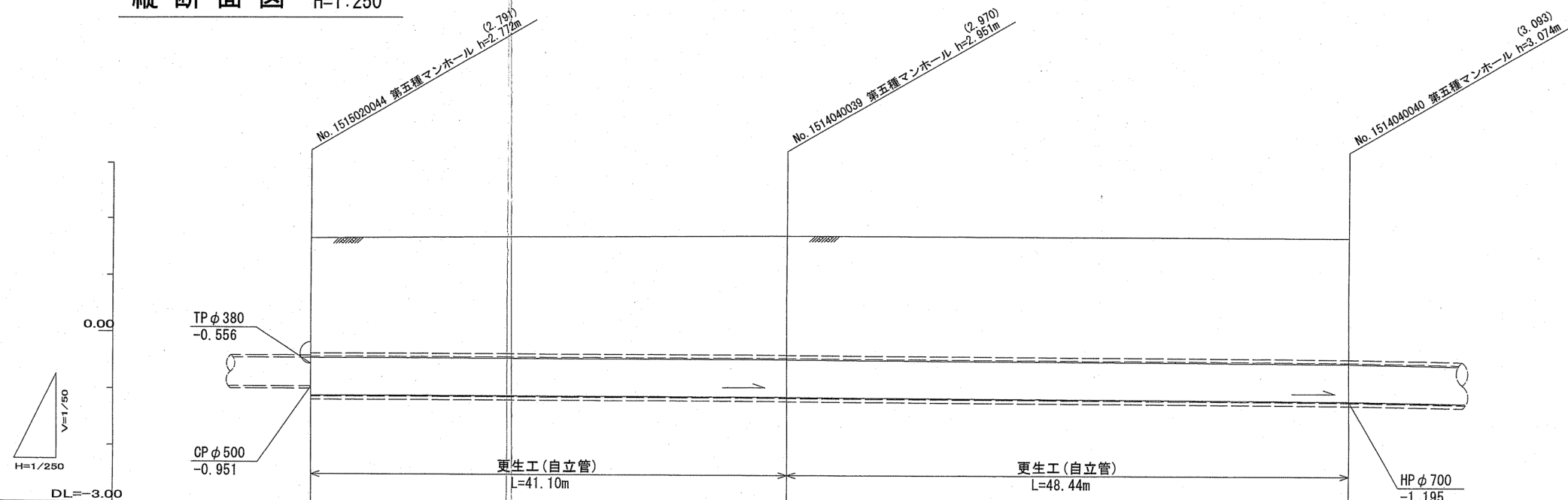
縦断面図 V=1:50 H=1:250
