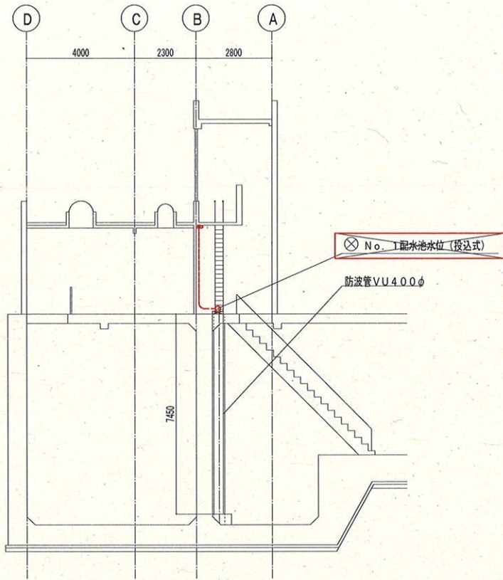
断面図 S=1/200
