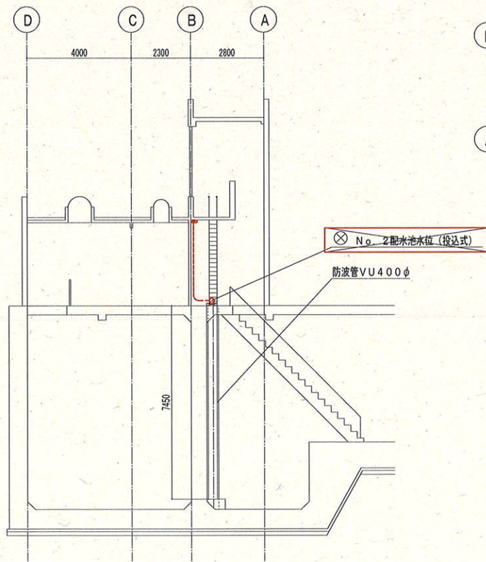
断面図 S=1/200
