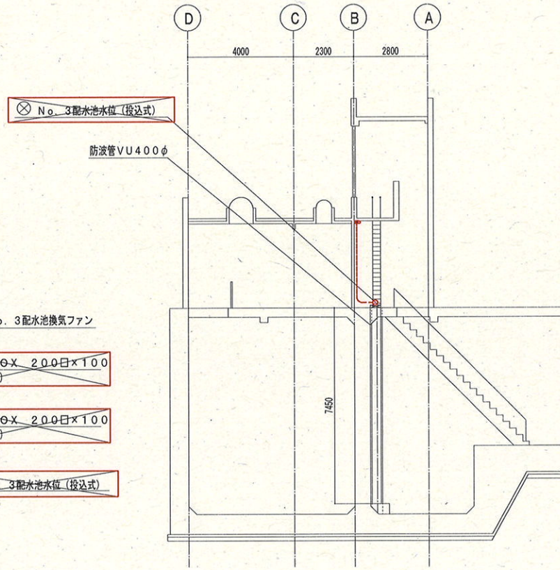
断面図 S=1/200
