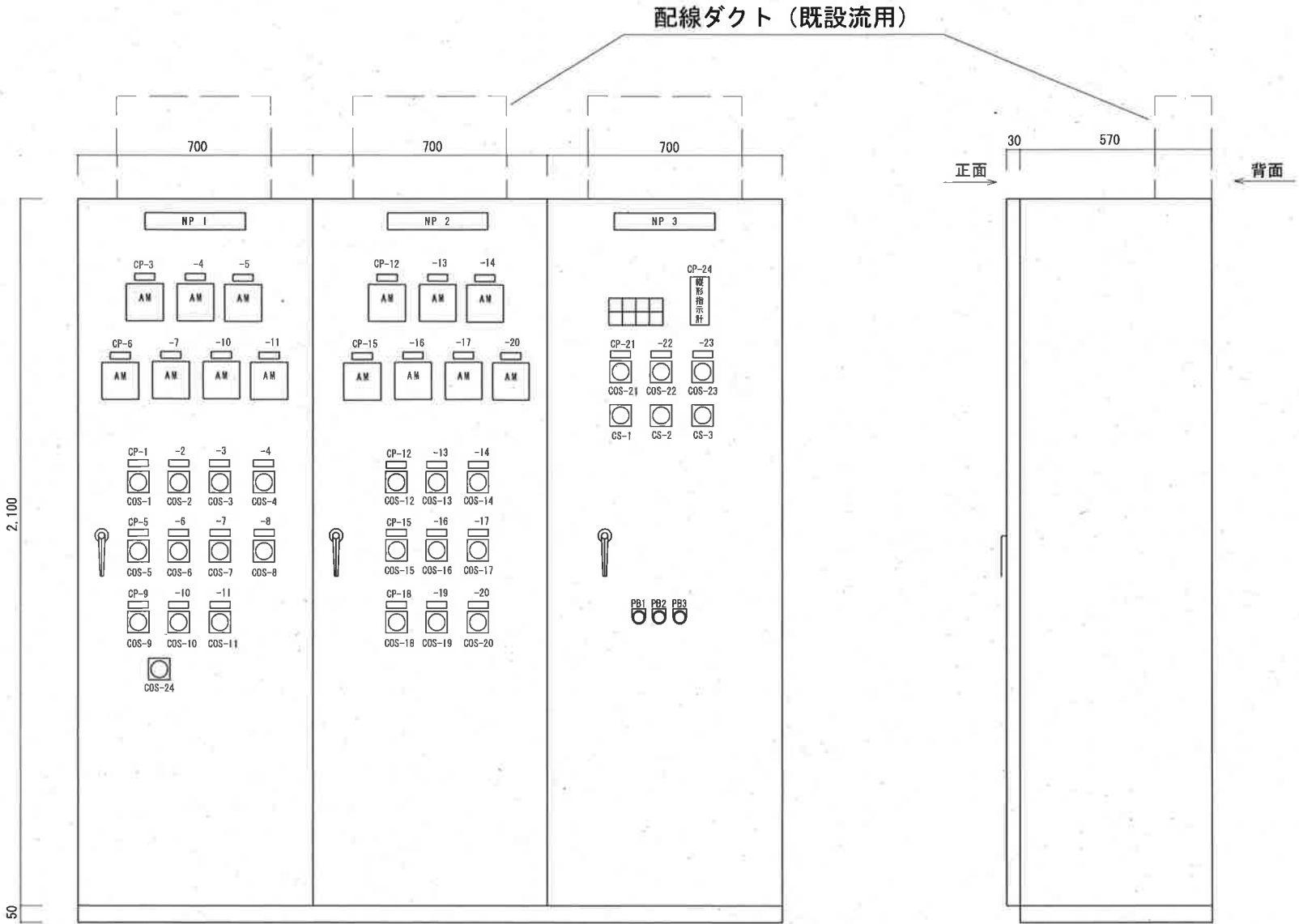
正面図
