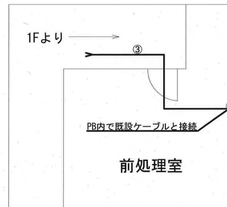
B1F平面図
