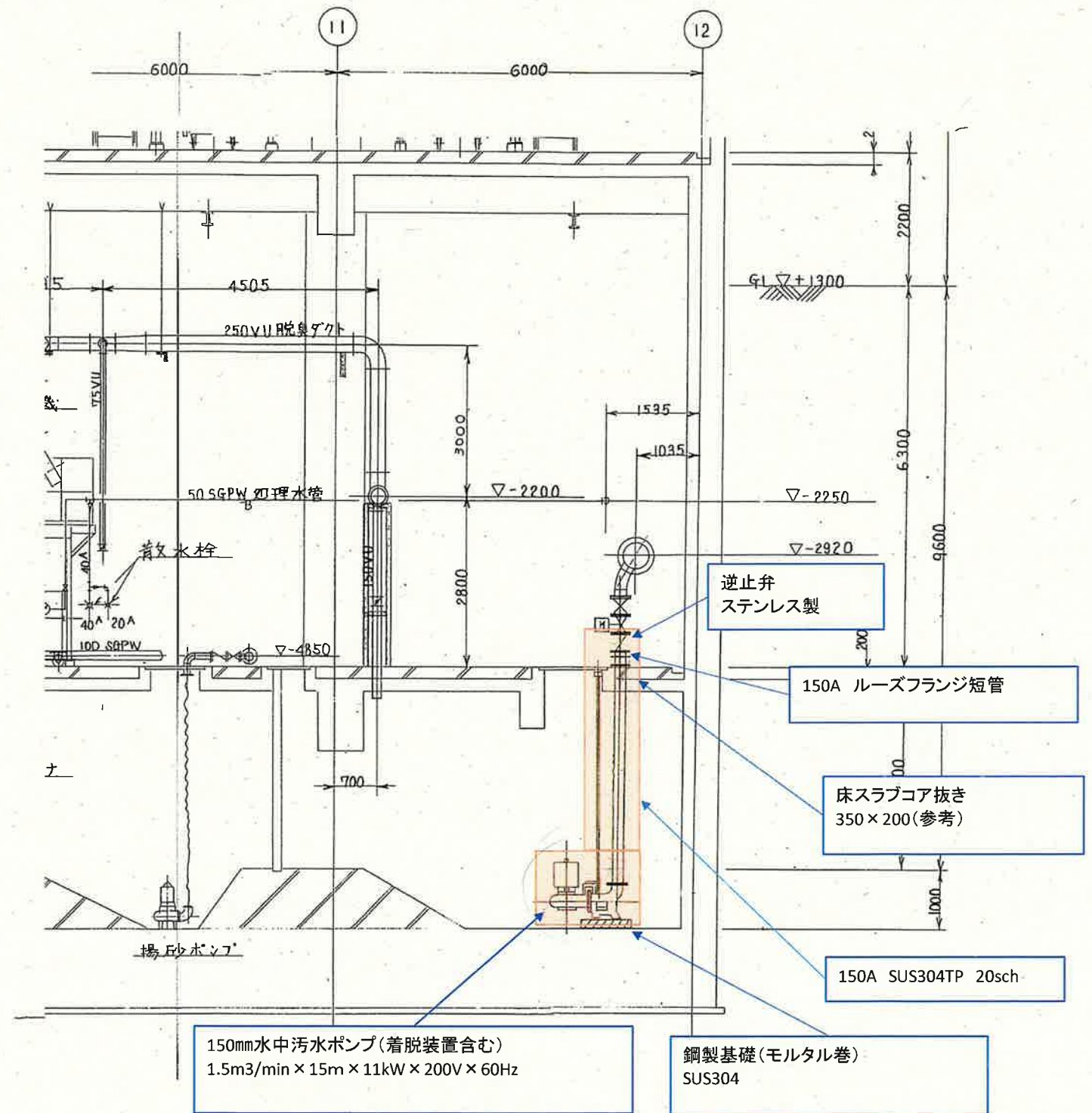
更新後 沈砂池, 地下二階断面図
