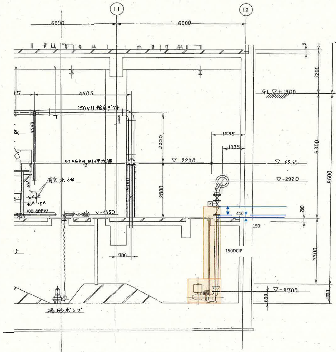
更新前 沈砂池, 地下二階断面図
