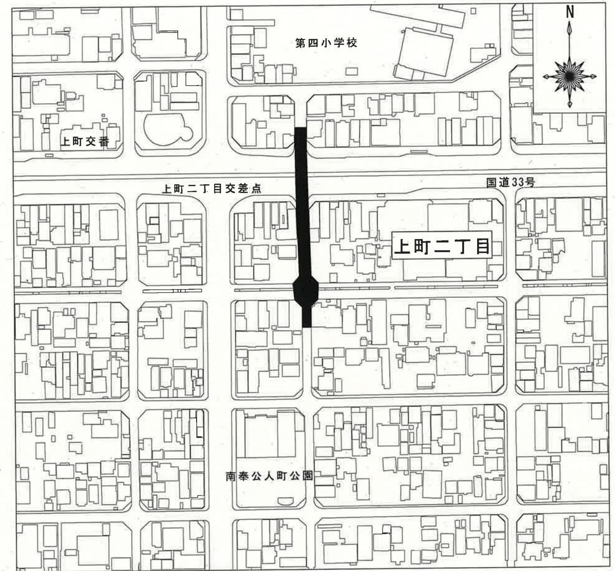
位置図 S=1:2500
