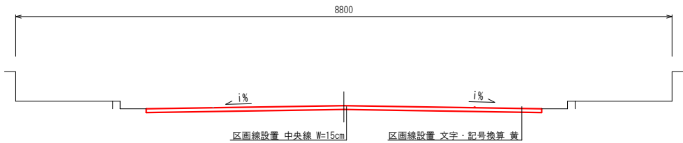
標準断面図 S=1:50
