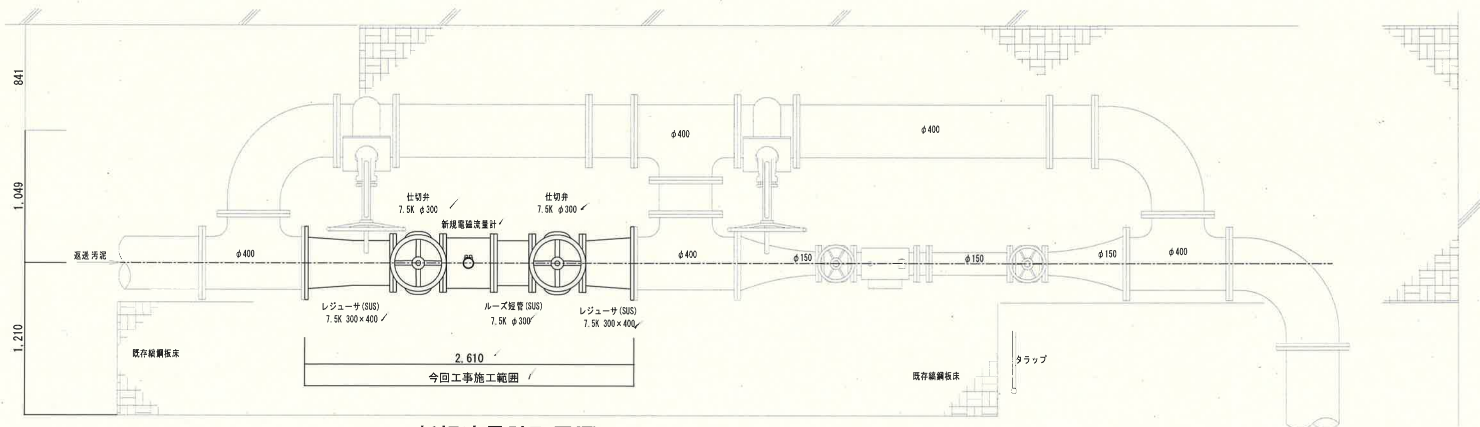
新規模流量計配置図
