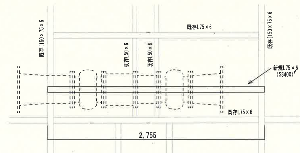
床面補強配置図 (A-A矢視図)
