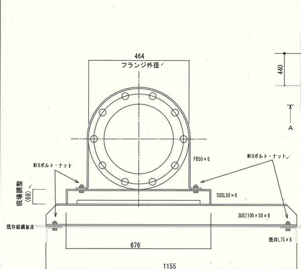
支持架台詳細図(1:10)
