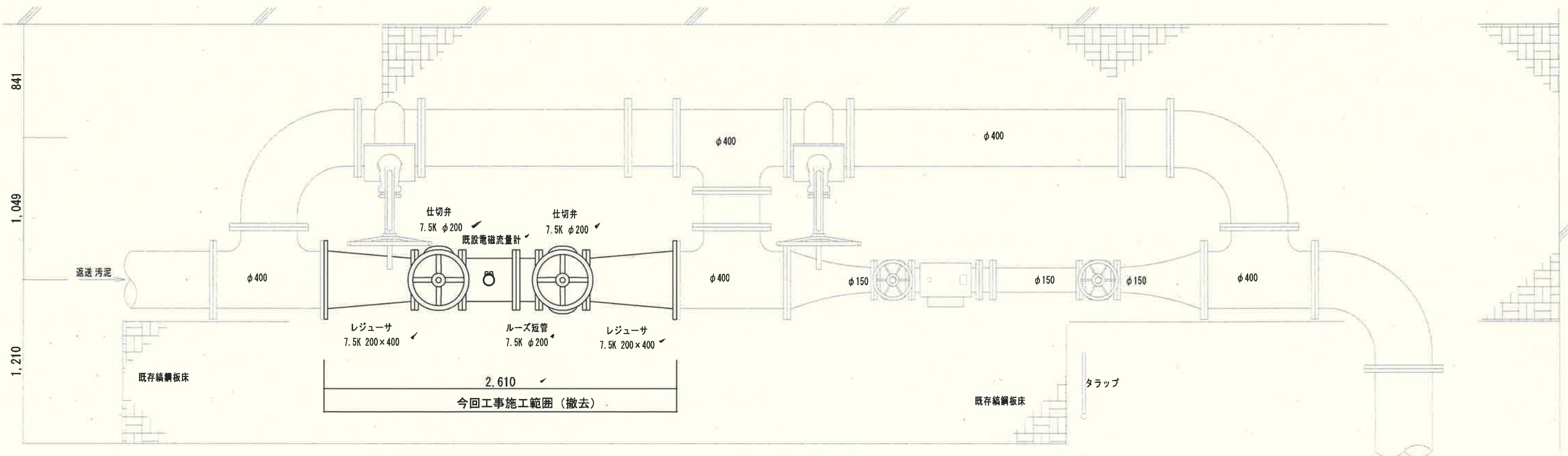
既設流量計配置図
