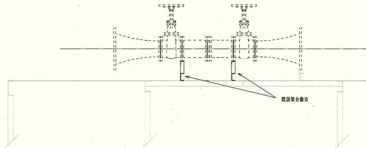
既設支持架台配置図
