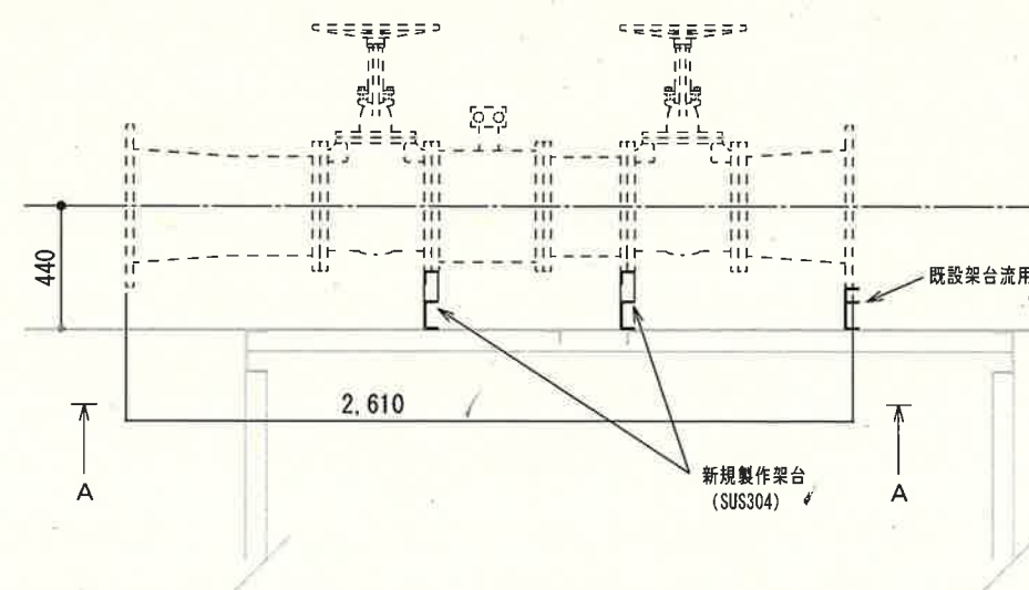
支持架台配置図
