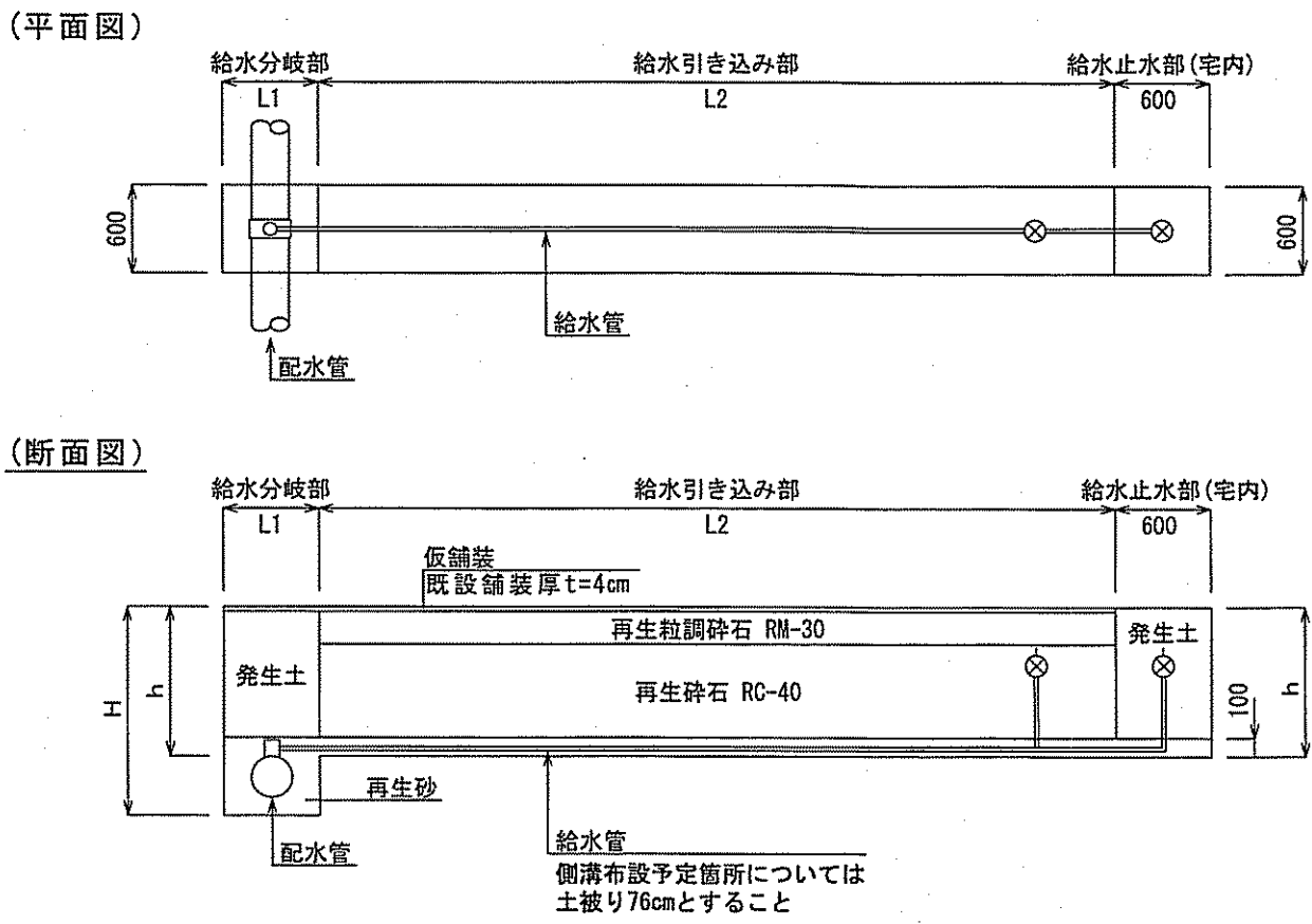
給水切替標準図 S=Free
