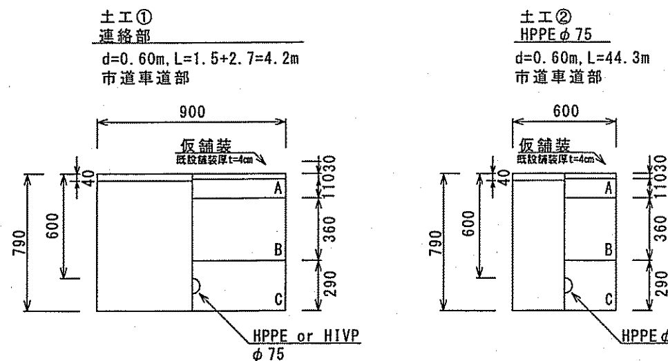
土工断面図 S=1:30
