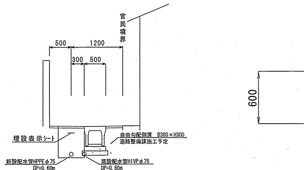
横断面図 S=1/50
