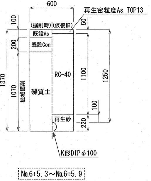
K形DIPφ100標準部
