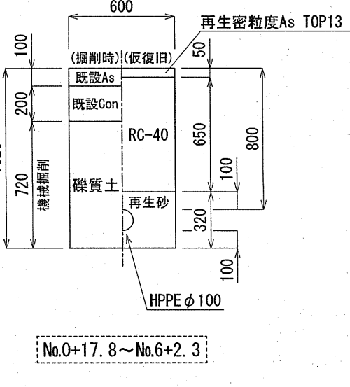
HPPEφ100標準部③
