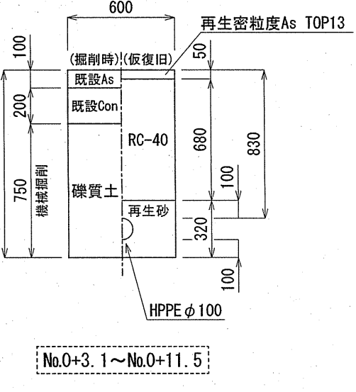
HPPEφ100標準部①
