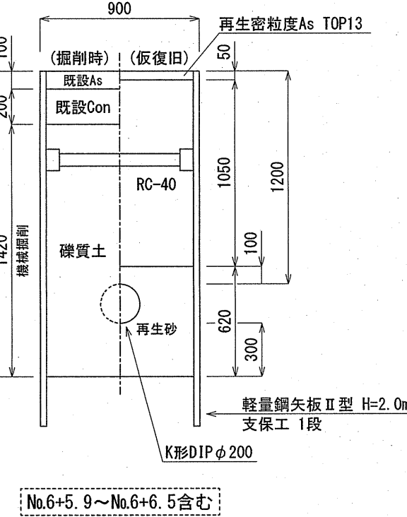
K形DIPφ200連絡部
