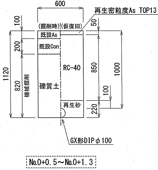
GX形DIPφ100標準部①
