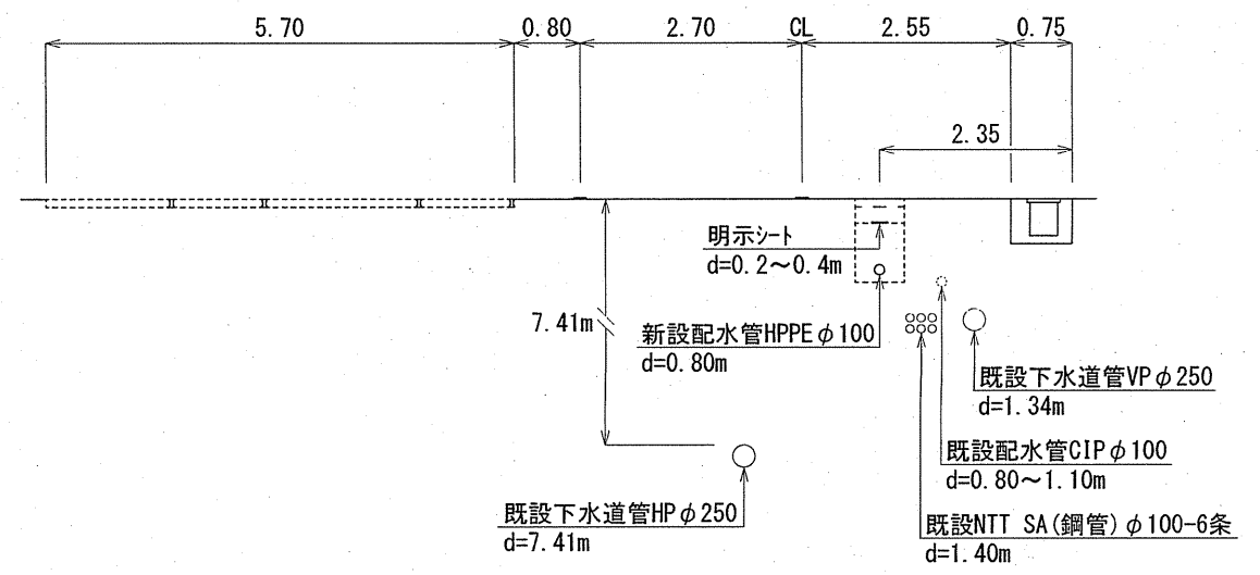
B-B' 横断面図 S=1:100
