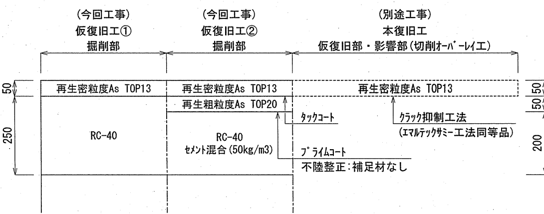
舗装構成図 S=Free
