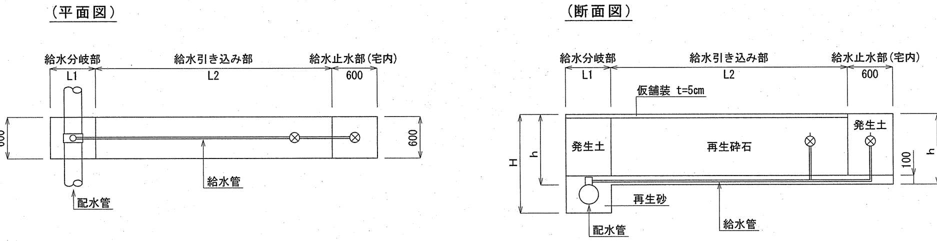
切替標準図 S=Free
