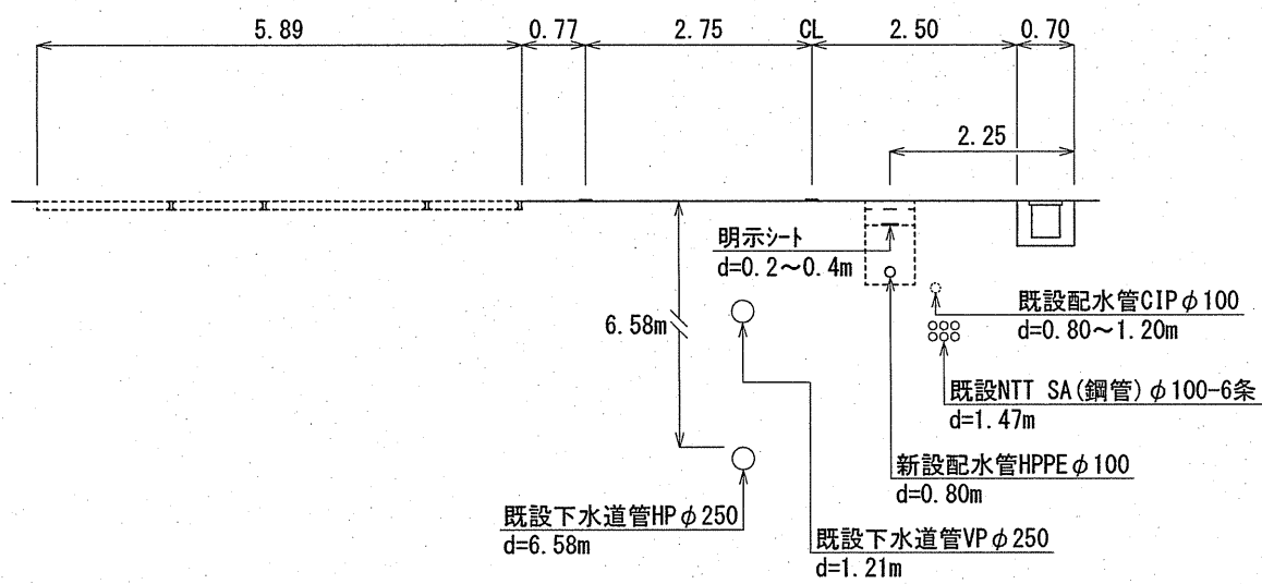
B-B' 横断面図 S=1:100
