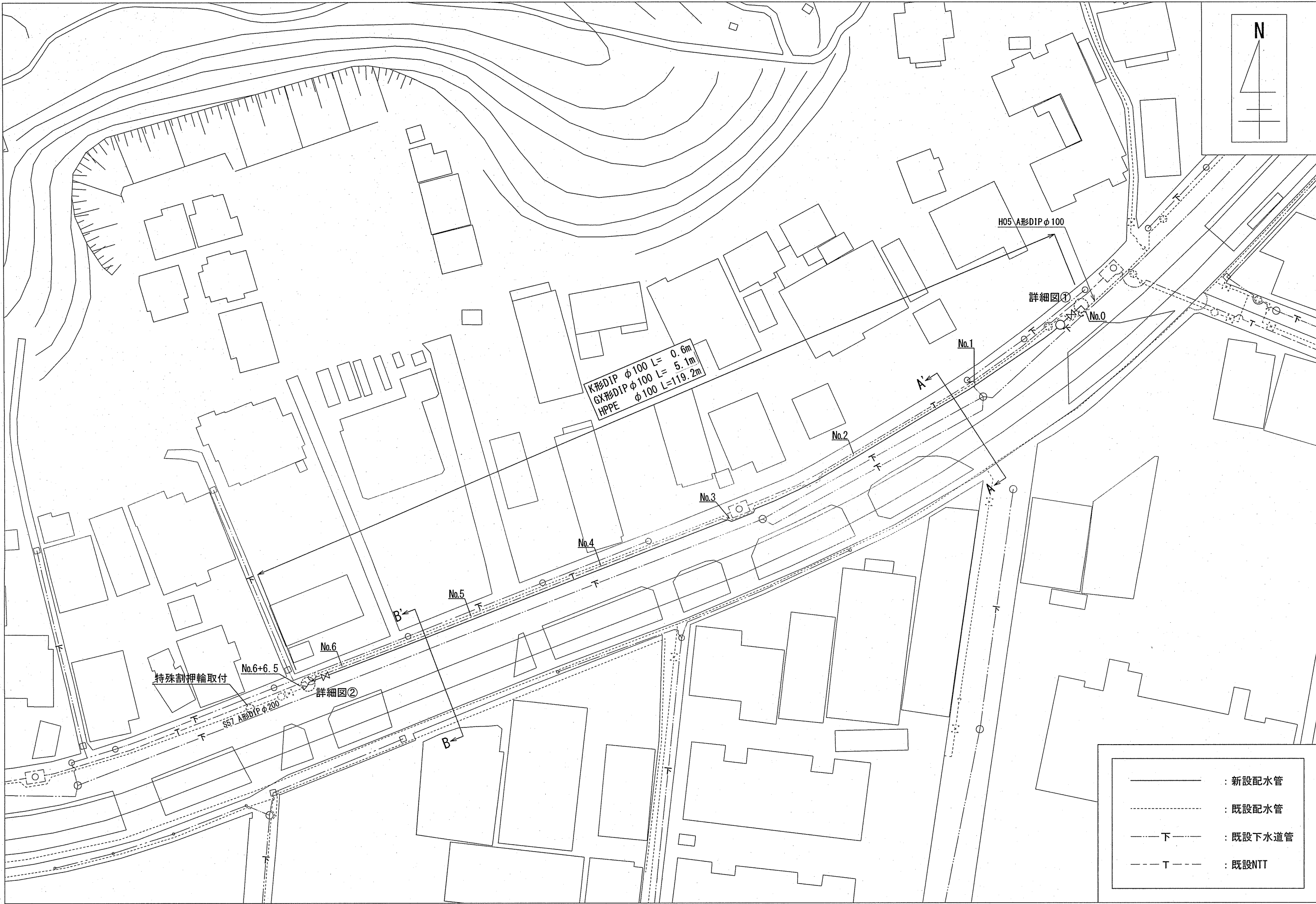
土工図 S=1:30
