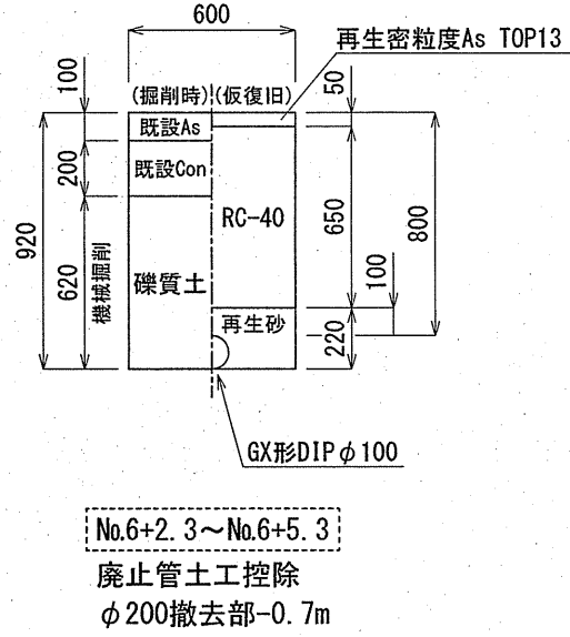
GX形DIPφ100標準部③
