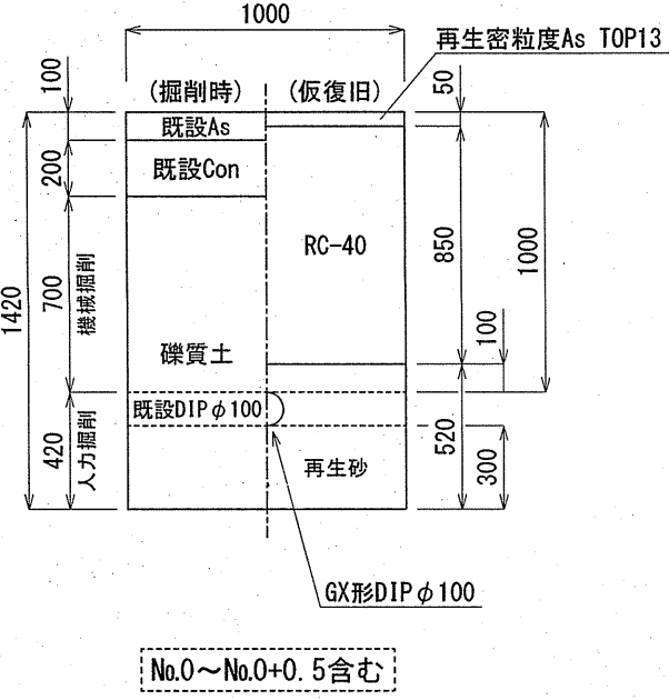
GX形DIPφ100標準部③
