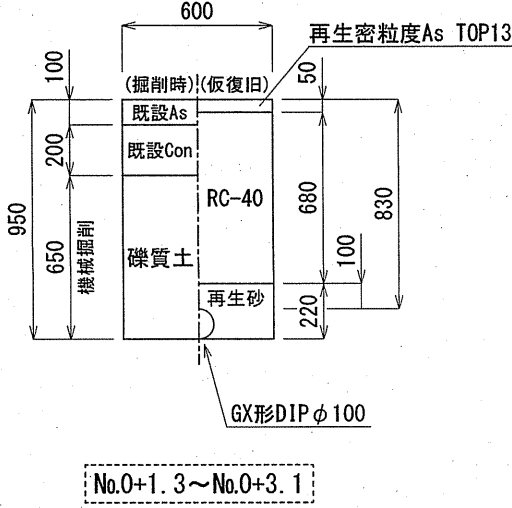
GX形DIPφ100標準部②
