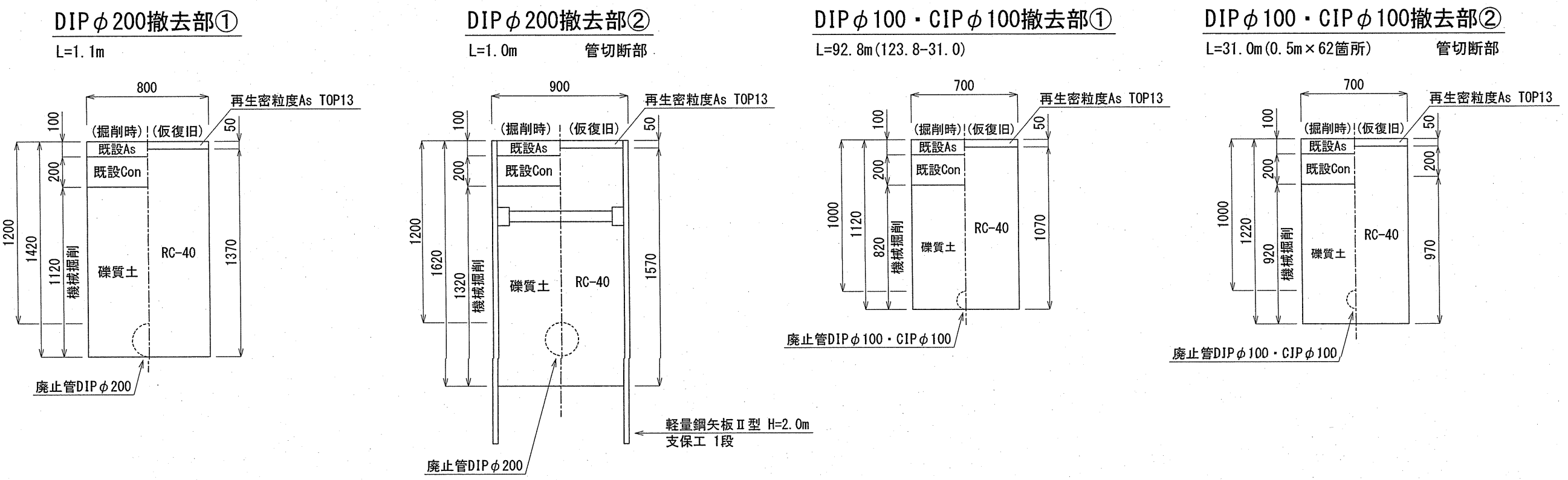
廃止管土工図 S=1:30
