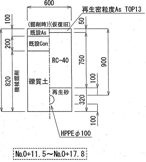
HPPEφ100標準部②
