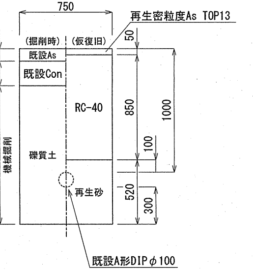
キャップ止施工部
