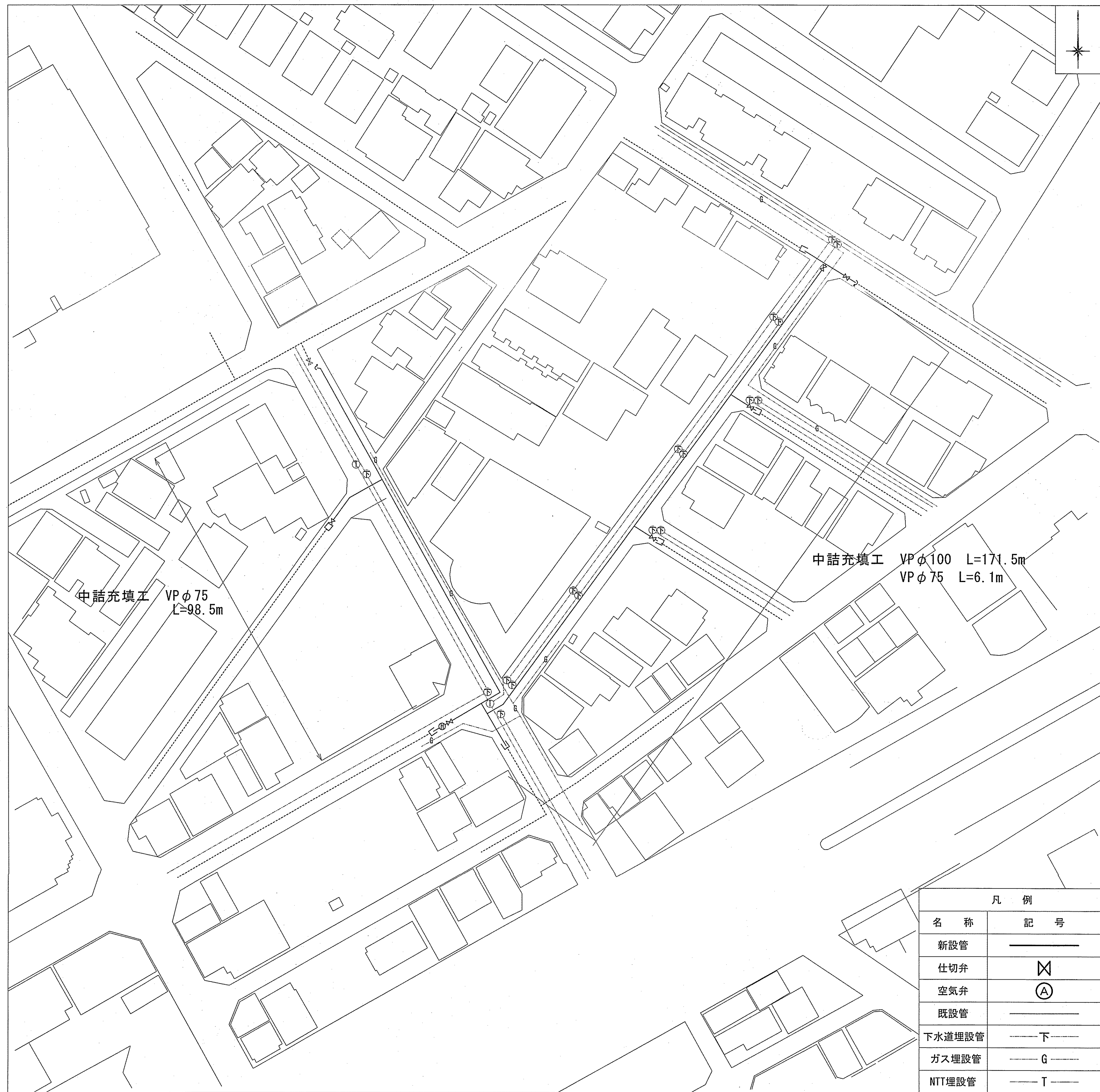
廃止管平面図 S=1:500
