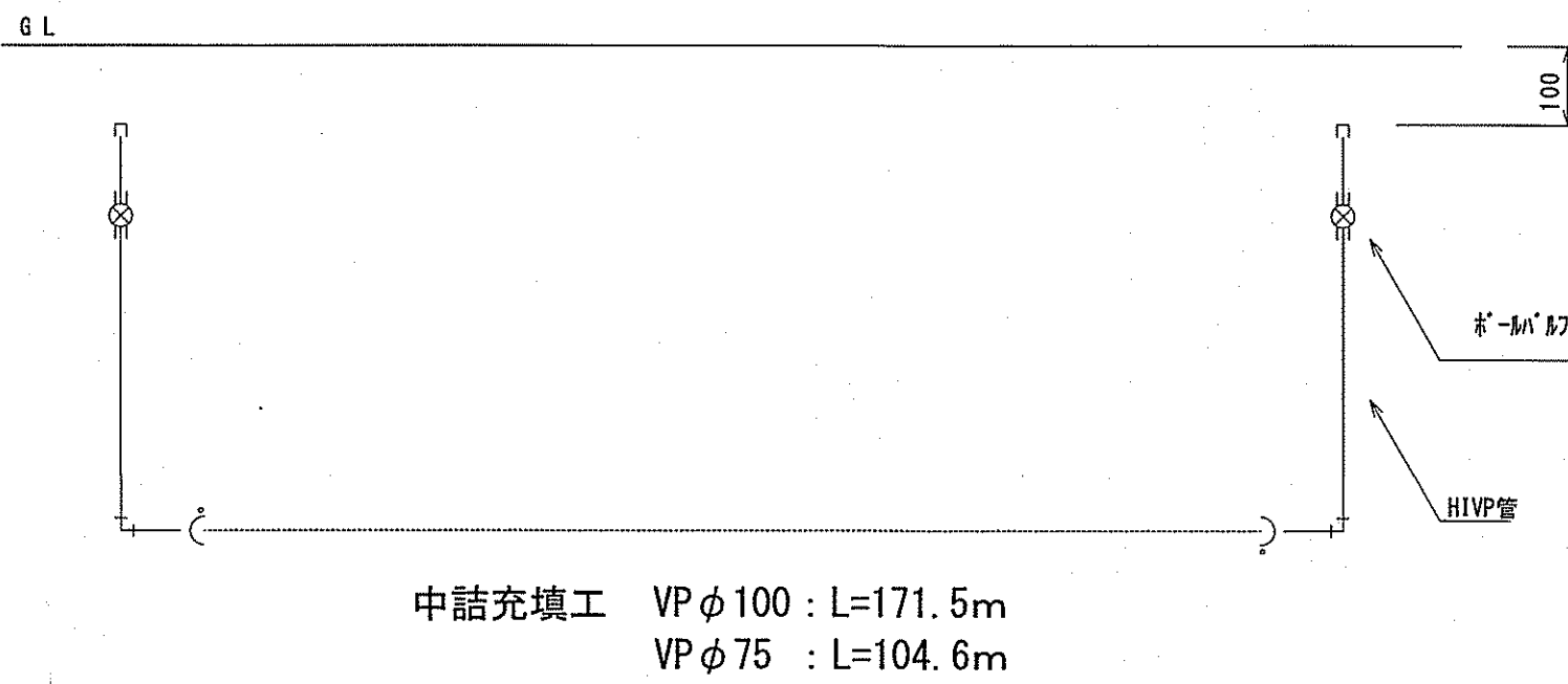
廃止管中詰充填図 S=FREE
