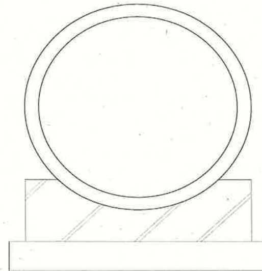
はつり調査箇所断面図
