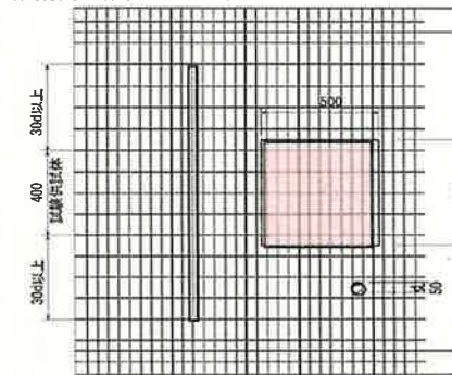
鉄筋採取に伴うはつり込み図
