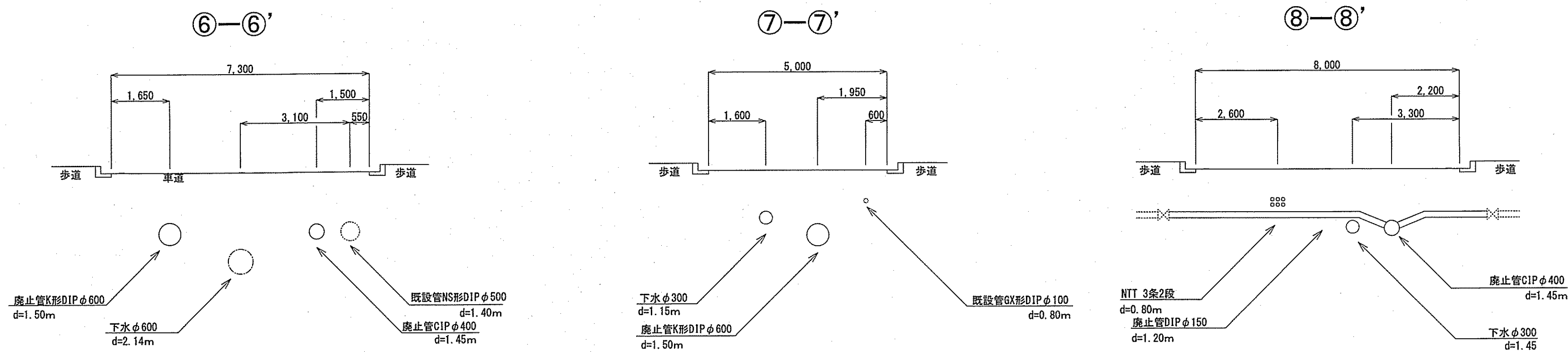
横断図(3) S=1:100
