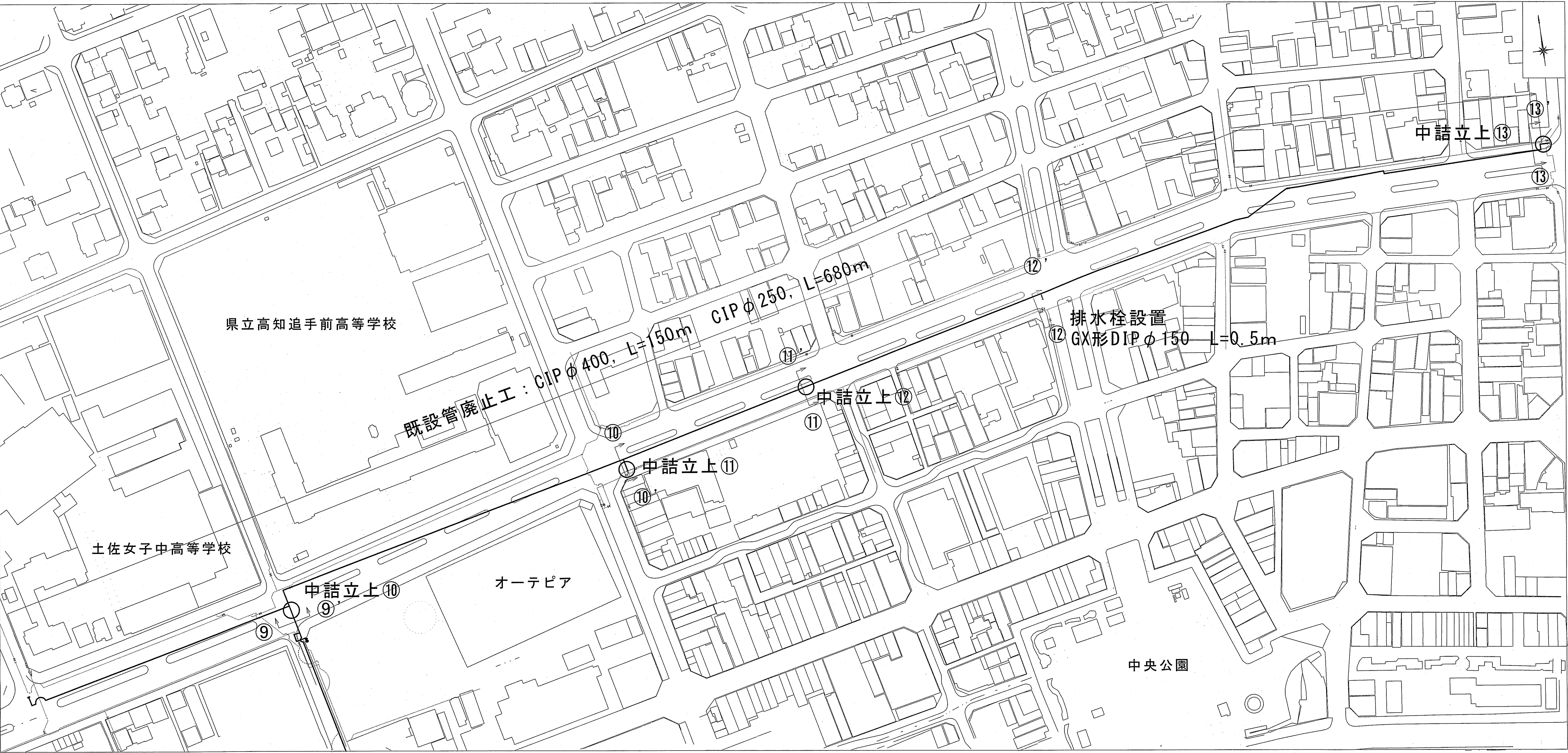
平面図(4) S=1:1000
