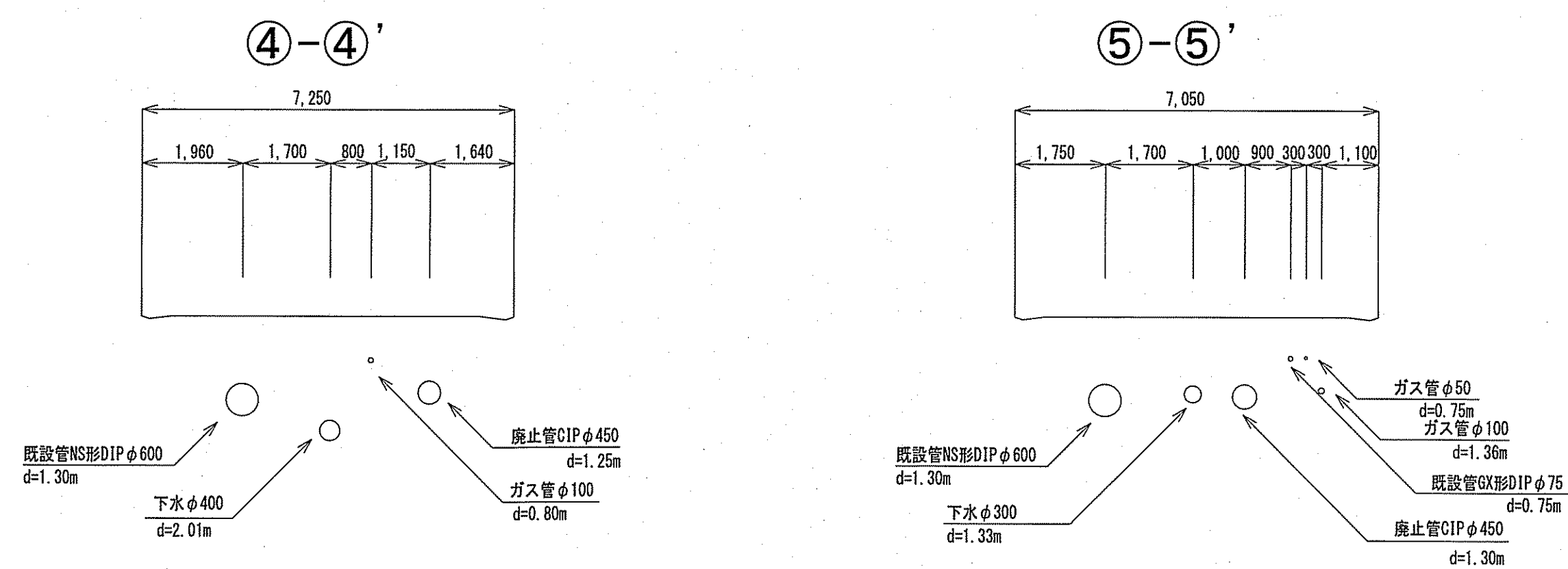
横断面図(2) S=1:100
