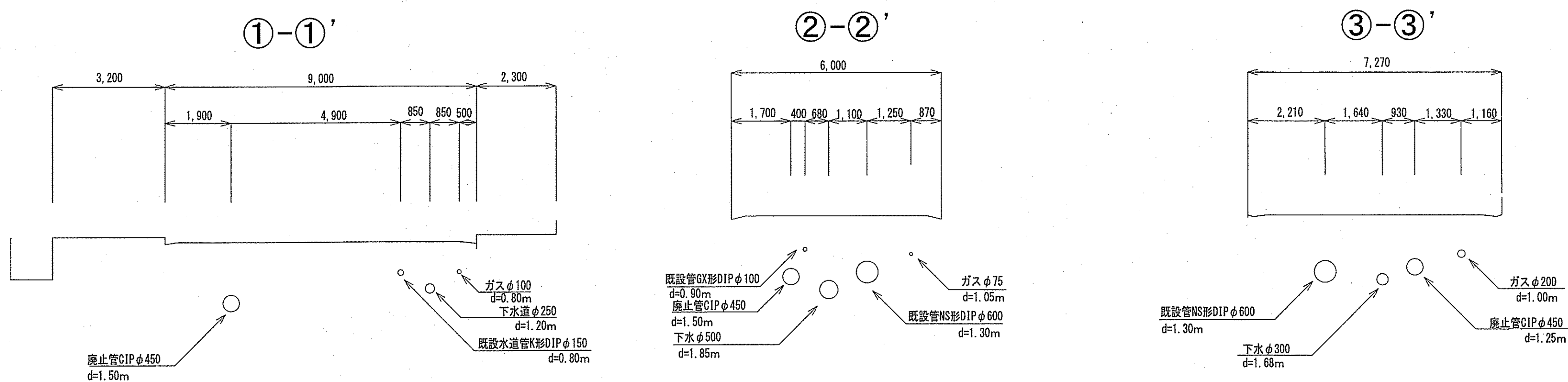
横断図(1) S=1:100
