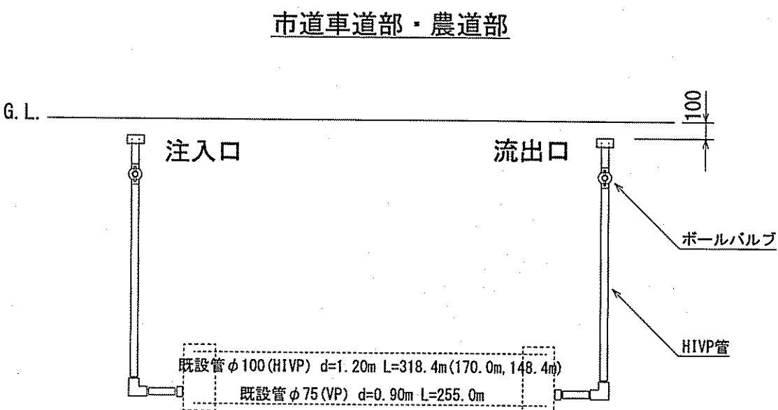
廃止管中詰充填図 S=1:Free
