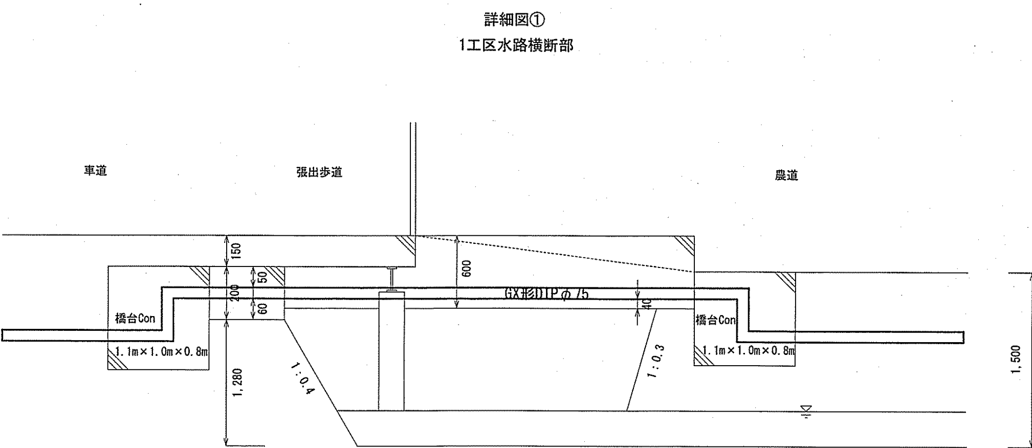
詳細図 S=1:Free
