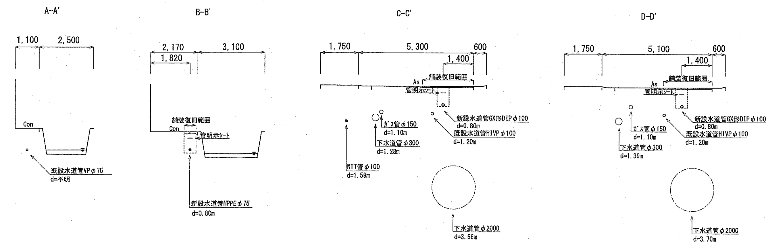
詳細図 S=1:Free
