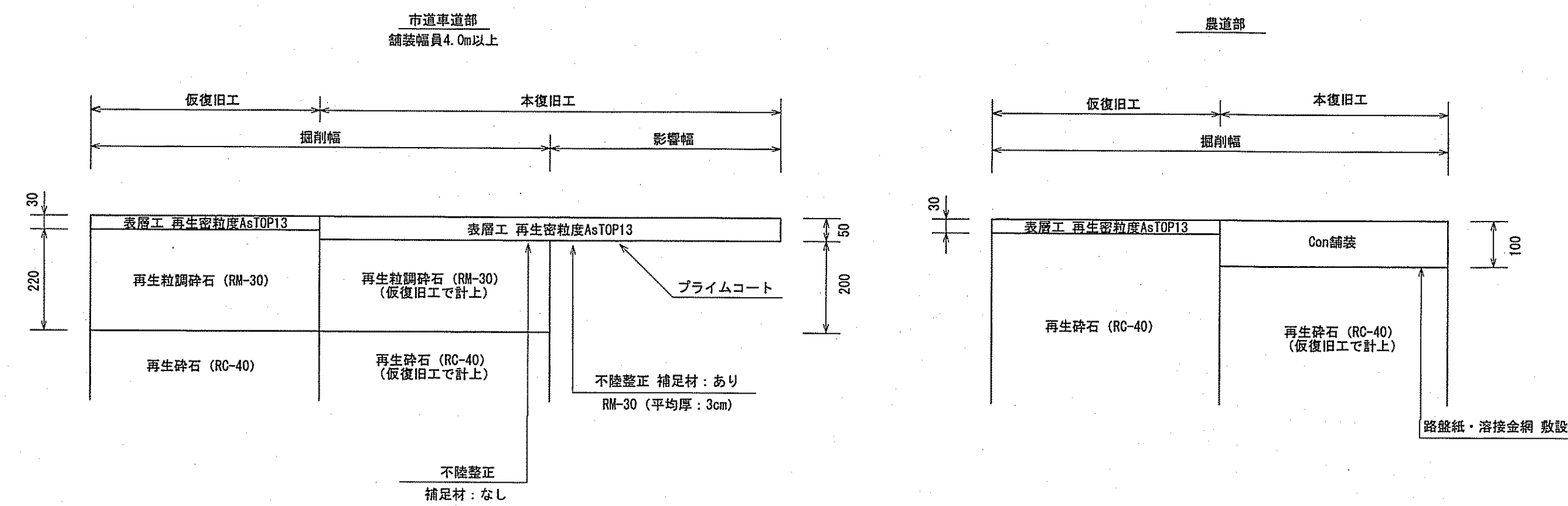
舗装復旧断面図 S=1:10
