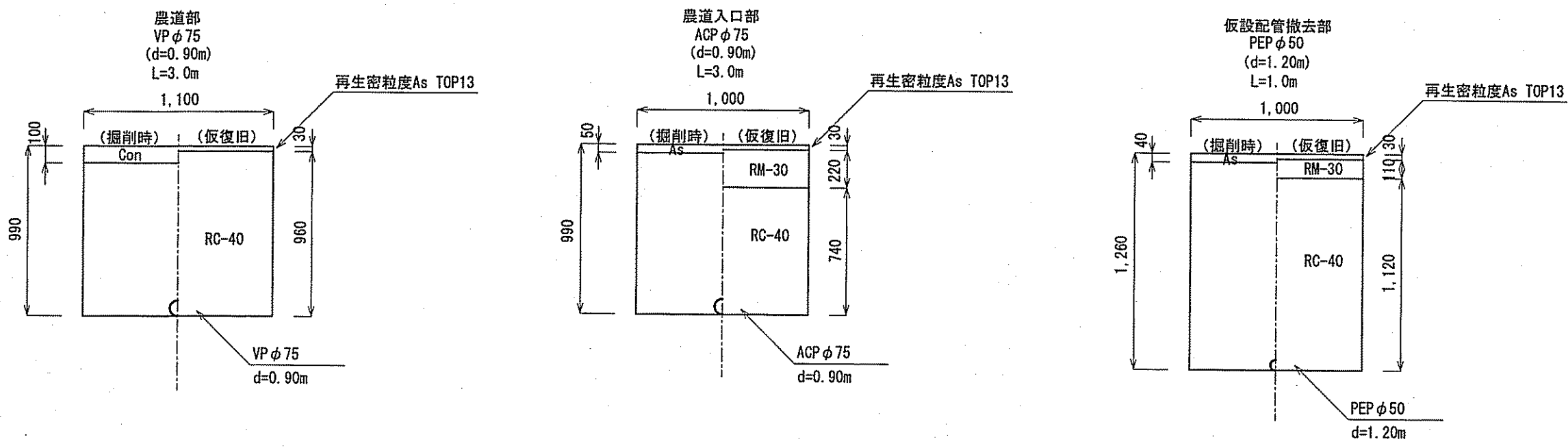
廃止管土工断面図 S=1:30
