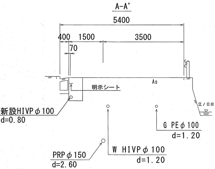
横断図 S=1 : 50
