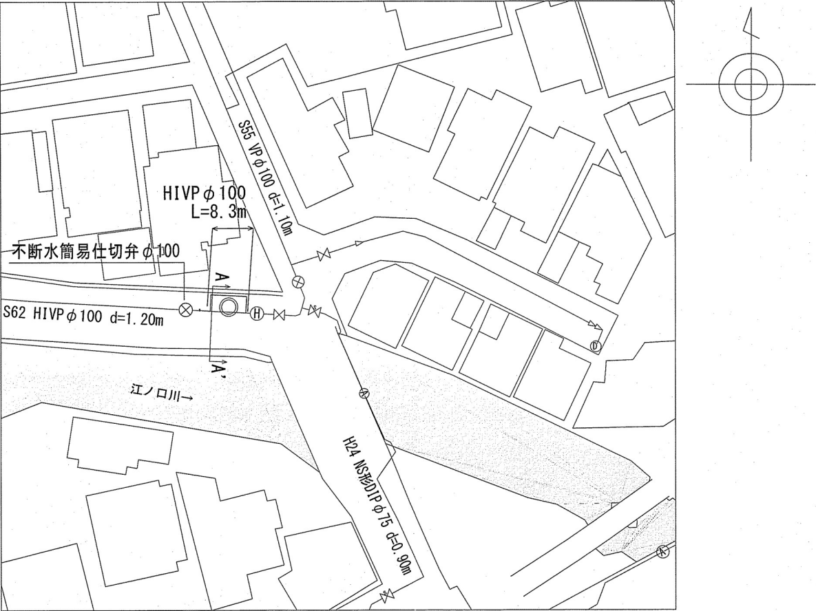
平面図 S=1 : 250
