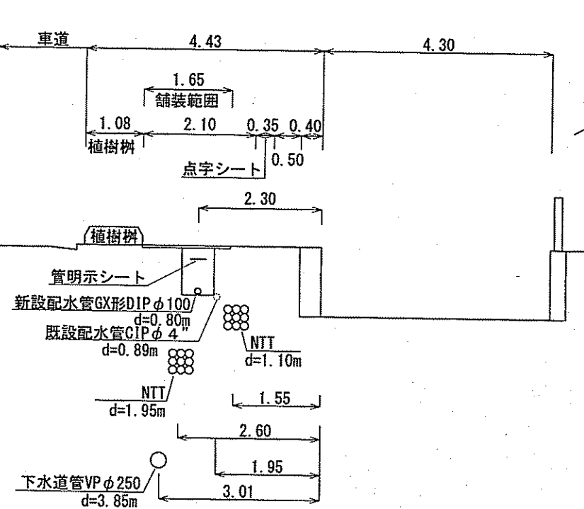
②-②' 横断面 S=1:100
