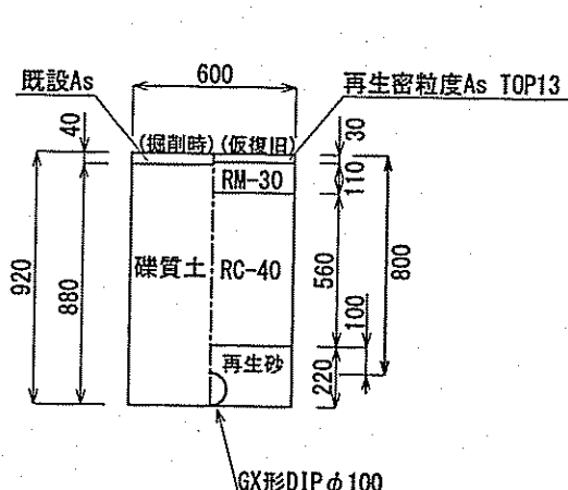
GXDIP φ100標準部①
