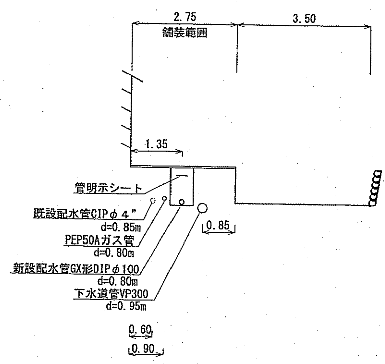
①-①' 横断面 S=1:100
