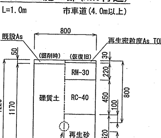
キャップ止施工部 (No.0付近)
