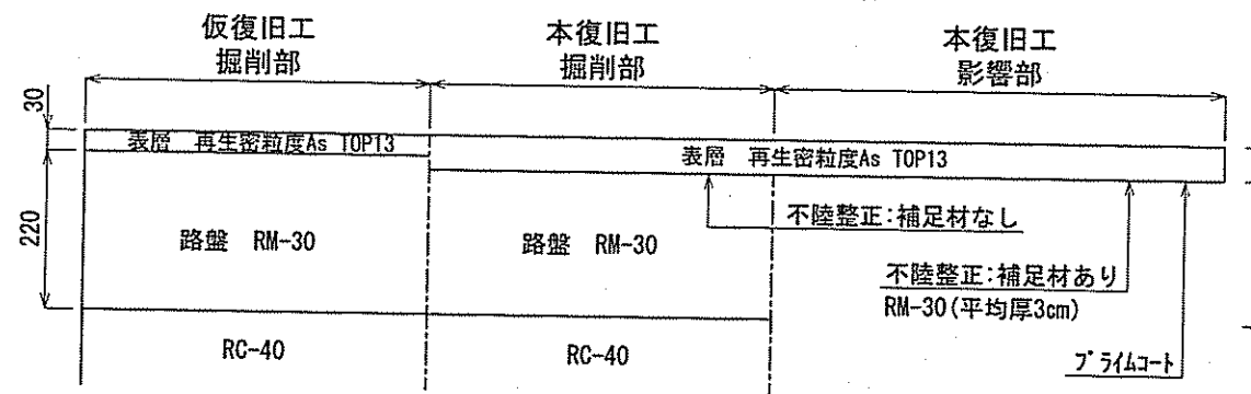
市道車道部 (As舗装)
