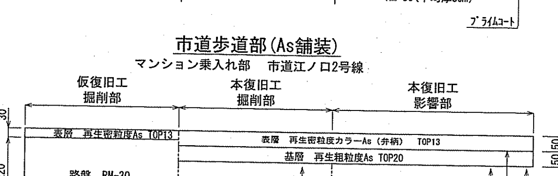
市道歩道部 (As舗装)
