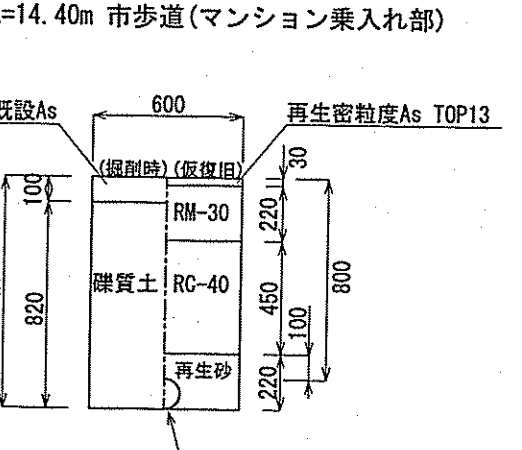
GXDIP φ100標準部⑤
