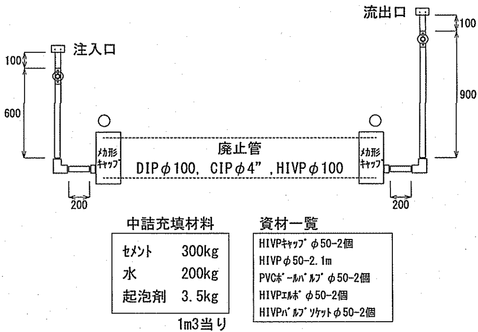
中詰充填工詳細図 S=Free 廃止管 L=195.3m
