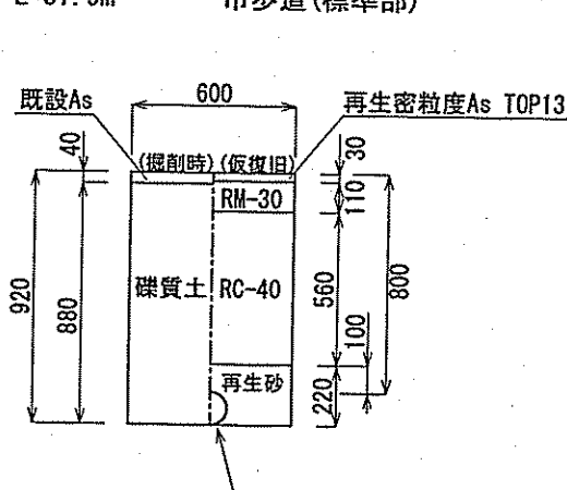
GXDIP φ100標準部③
