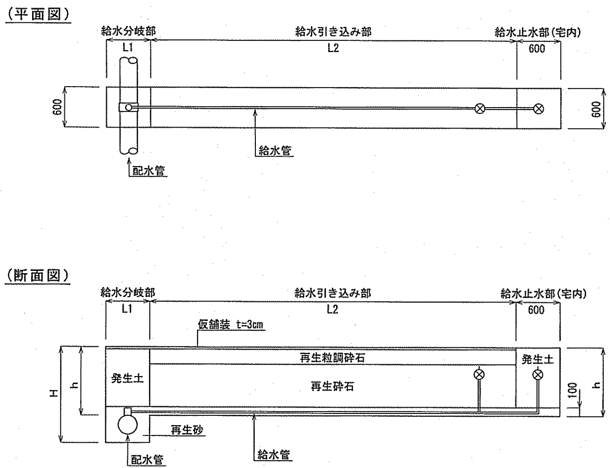
切替標準図 S=Free
