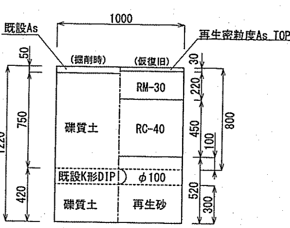
割字管取付部
