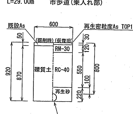
GXDIP φ100標準部④
