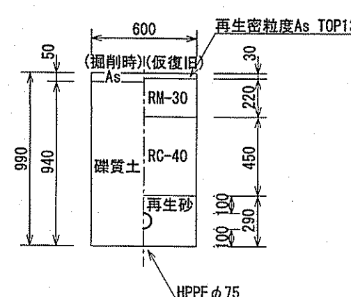
土工図④ HPPEφ75市道車道部 (d=0.80m) L=1.4m
