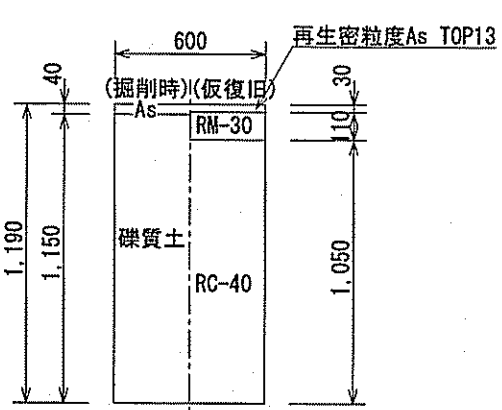
土工図⑪ 既設管廃止土工 (流出口②) L=1.5m
