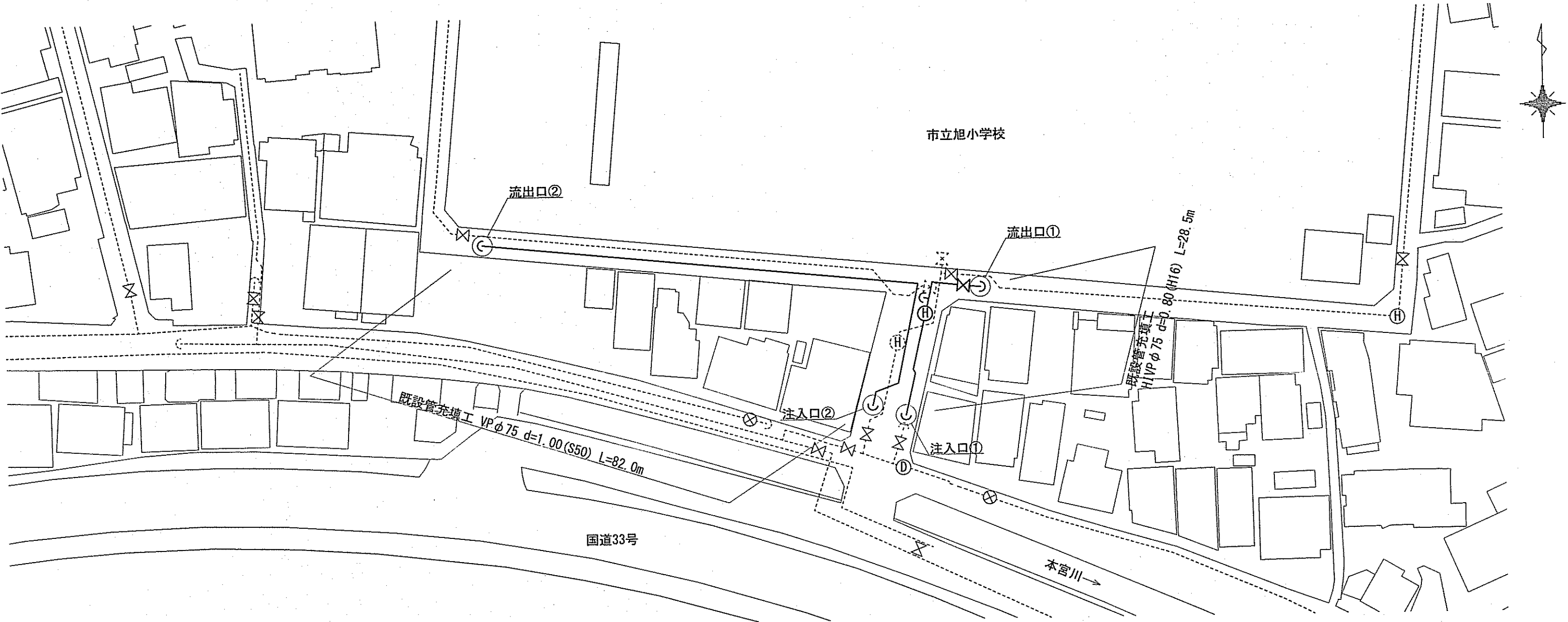
既設管廃止図 S=1/500
