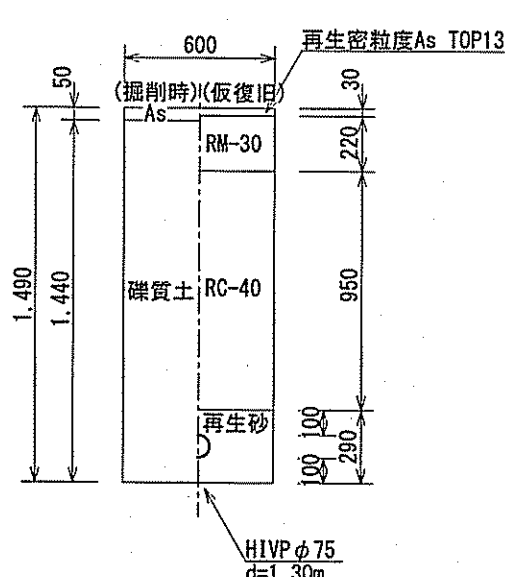
土工図⑦ HIVPφ75連絡部 (d=1.30m) L=1.9m
