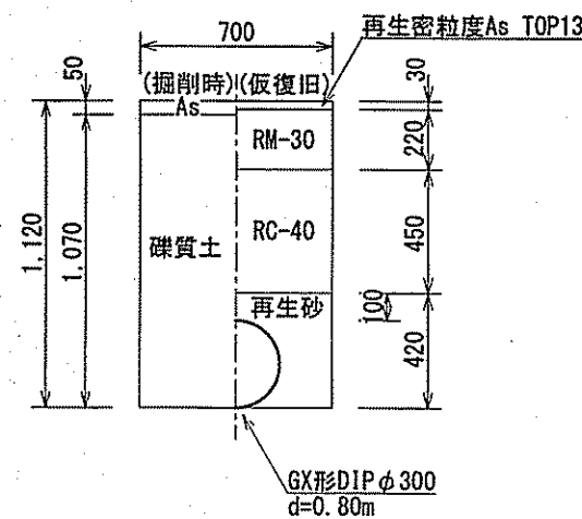
土工図① GX形DIPφ300市道車道部 (d=0.80m) L=8.6m
