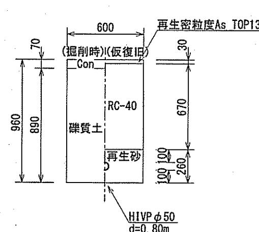
土工図⑨ HIVPφ50連絡部 (d=0.80m) L=2.9m
