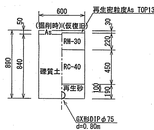
土工図③ GX形DIPφ75市道車道部 (d=0.80m) L=26.3m
