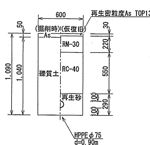
土工図⑧ HPPEφ75連絡部 (d=0.90m) L=2.0m
