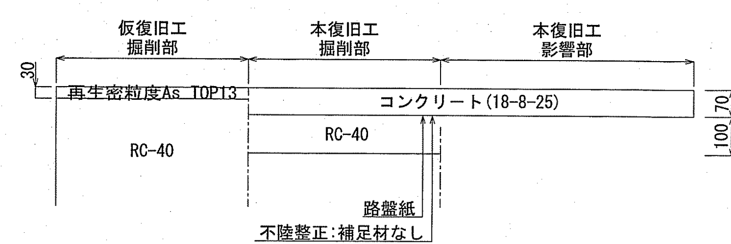
市道歩道部 (Con舗装)
