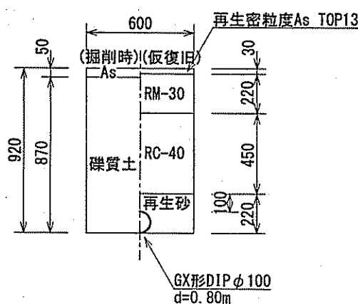
土工図② GX形DIPφ100市道車道部 (d=0.80m) L=3.6m
