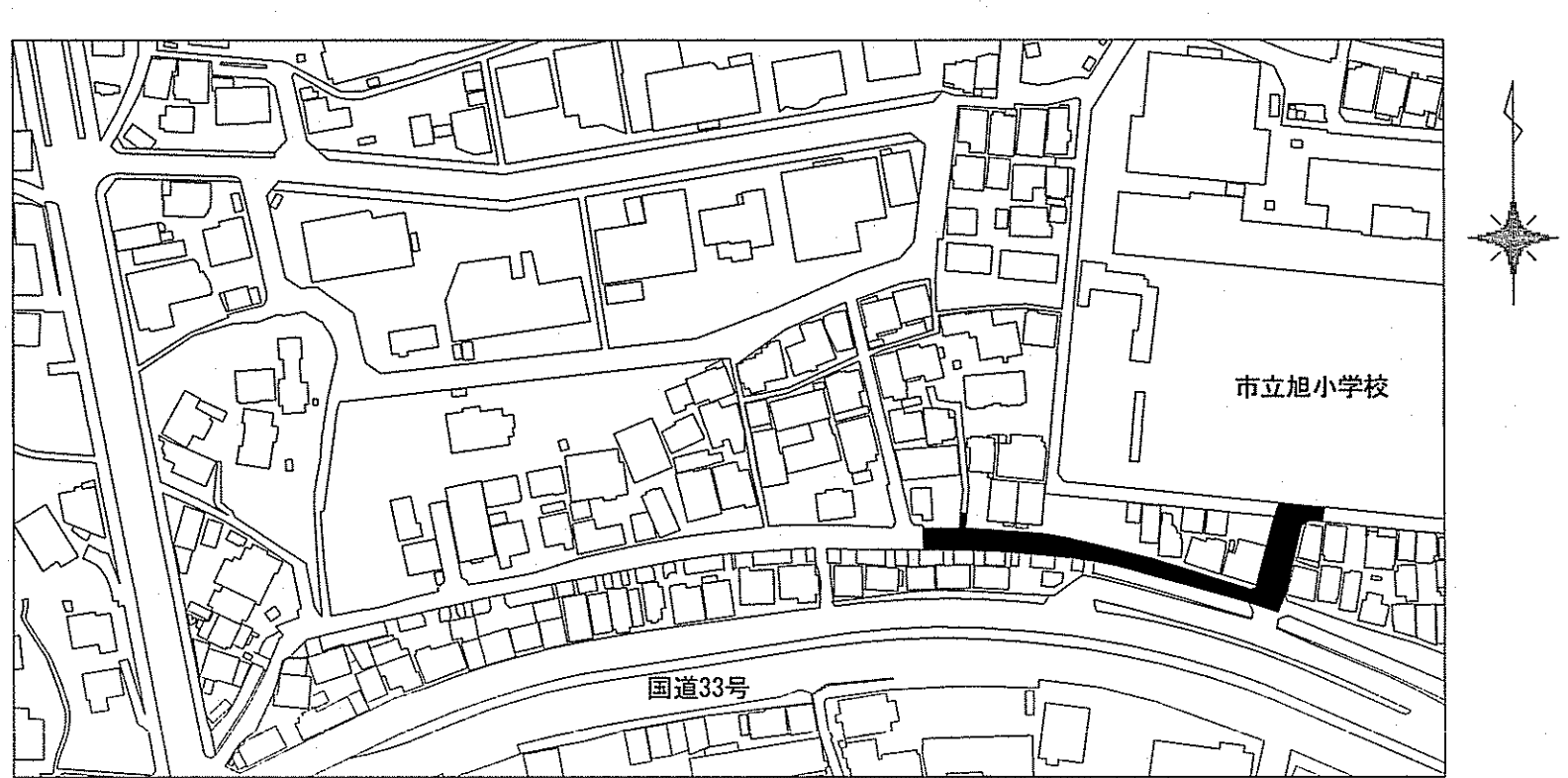
位置図 S=1/2,000
