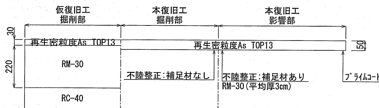
市道車道部 (As舗装) 舗装幅員4.0m以上
