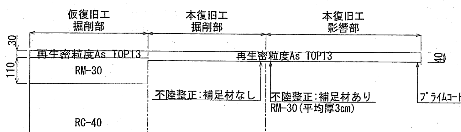
市道車道部 (As舗装) 舗装幅員4.0m未満
