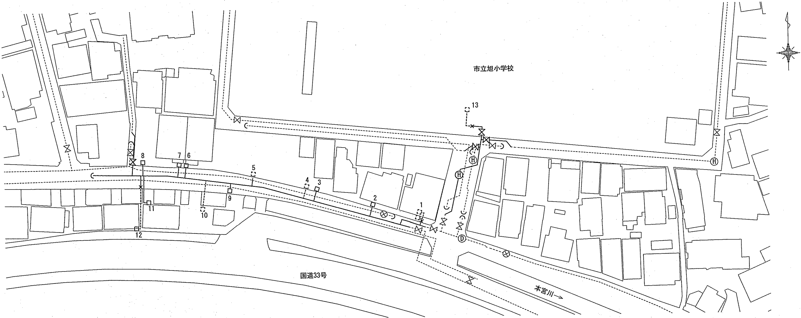
切替平面図 S=1/500
