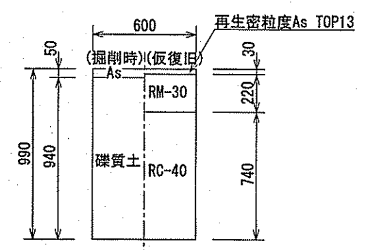
土工図⑩ 既設管廃止土工 (注入口①) L=1.5m
