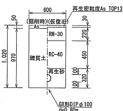
土工図⑥ GX形DIPφ100連絡部 (d=0.80m) L=2.4m
