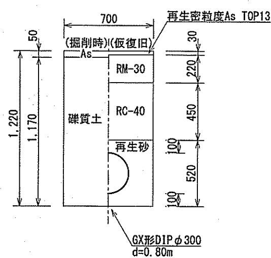
土工図⑤ GX形DIPφ300連絡部 (d=0.80m) L=1.0m
