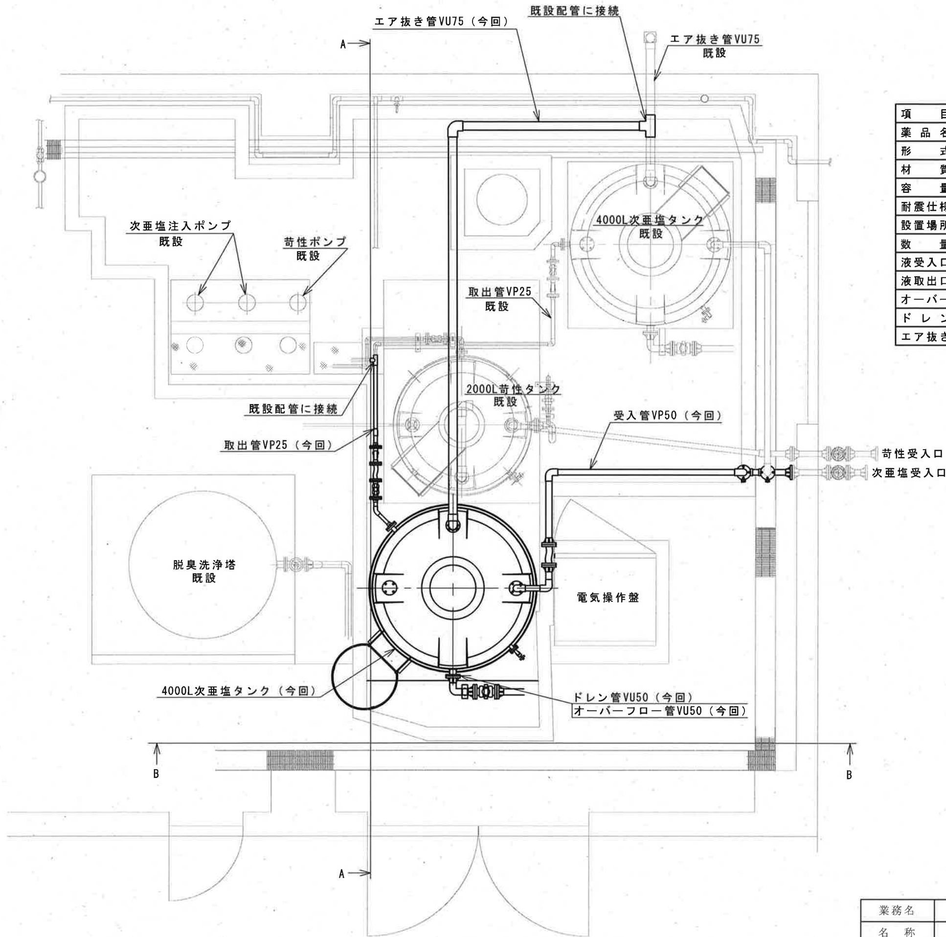
西処理場脱臭機棟平面図
