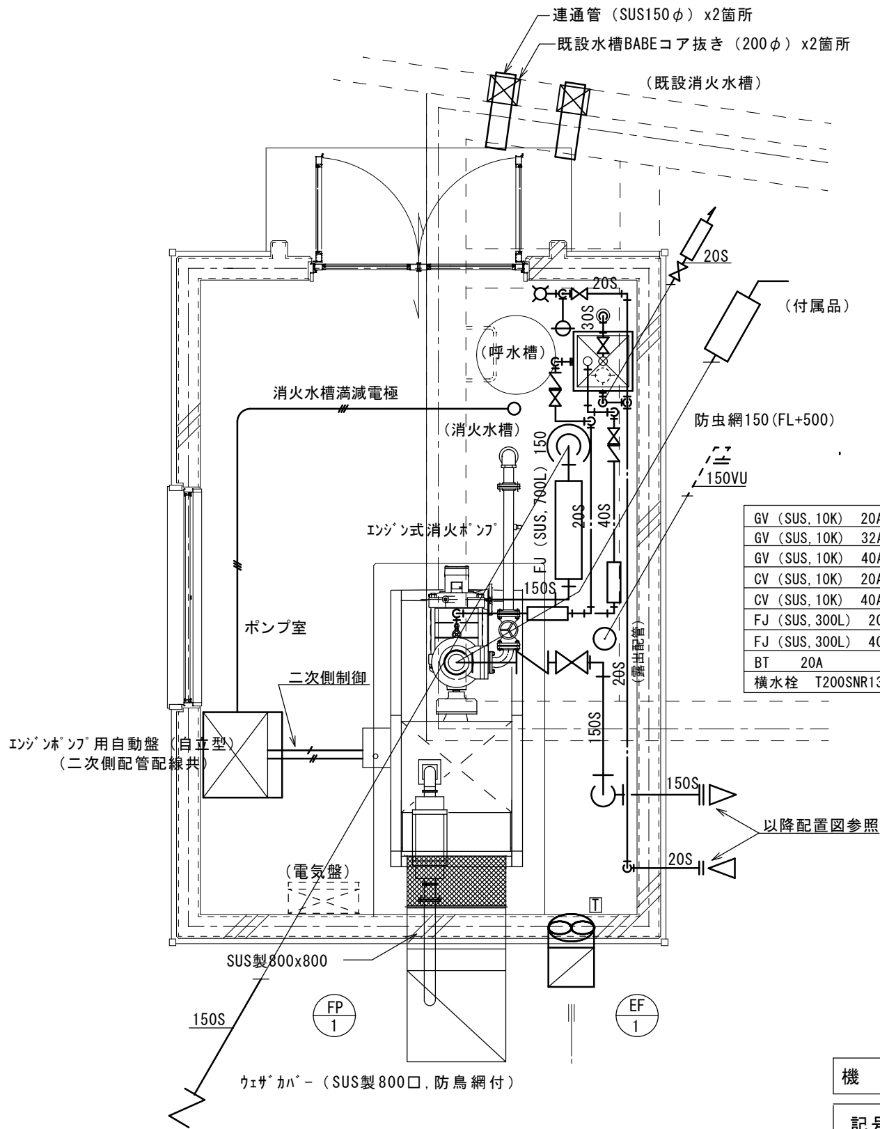
ポンプ室詳細図 1 / 4 0
