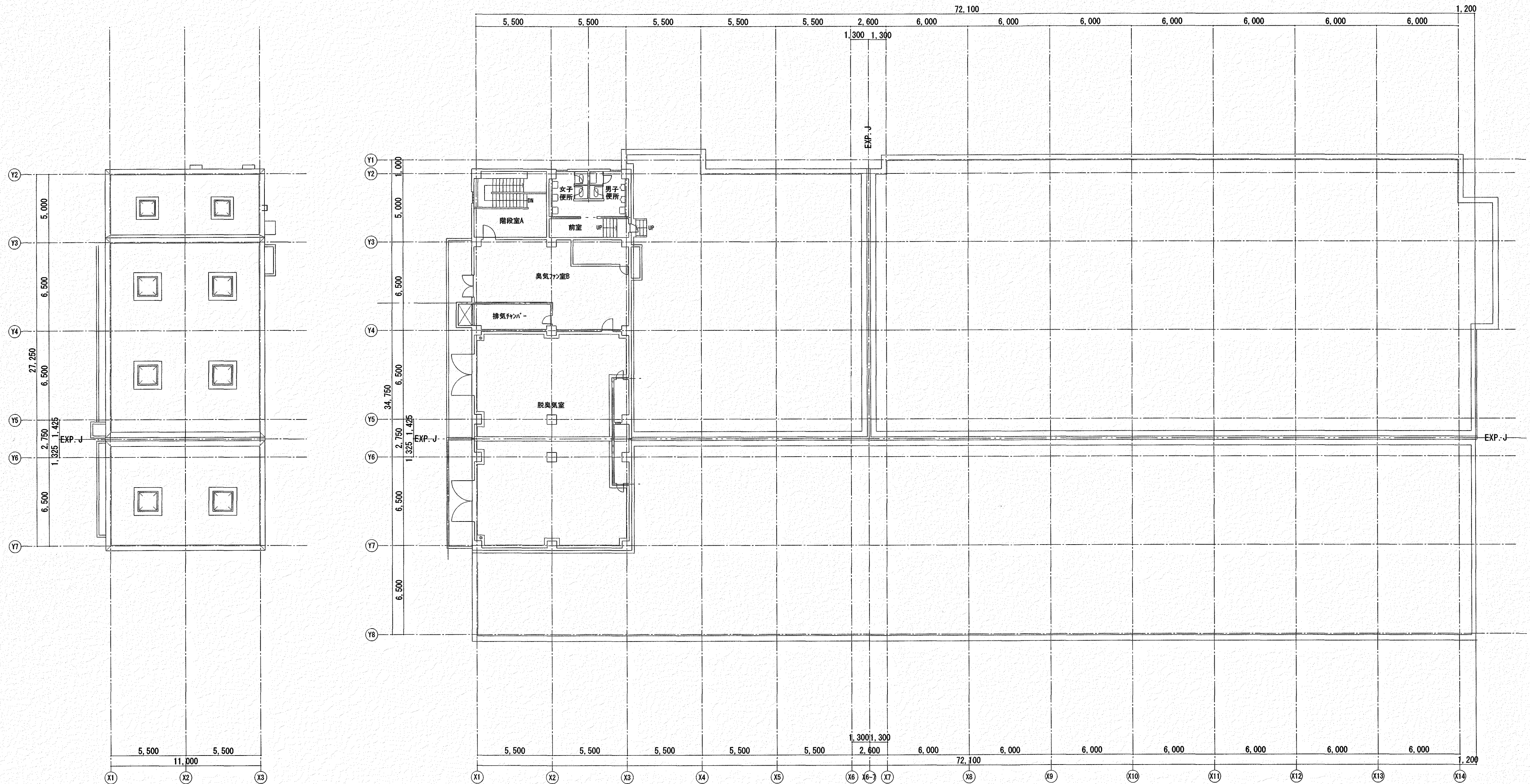
【水処理棟】2階平面図【参考図】 S=1/200
