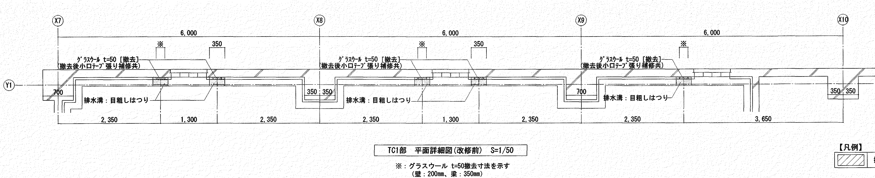
【水処理棟】TC1部 詳細図（改修前）
