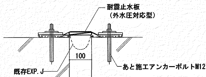
EXP. J部止水カバー詳細図 S=1:10
