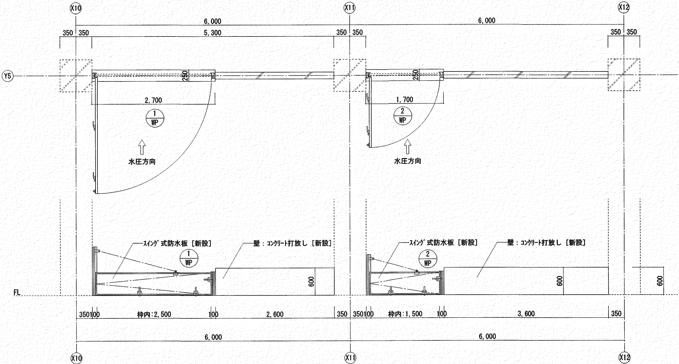
TW15部 平面詳細図(改修後) S=1/50
