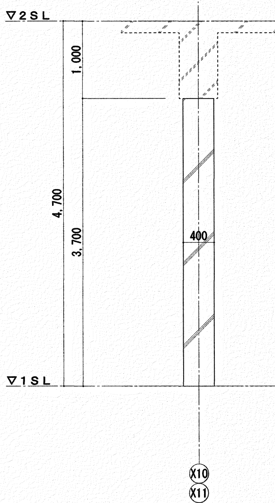
NW40A・B部 断面詳細図 S=1/50
