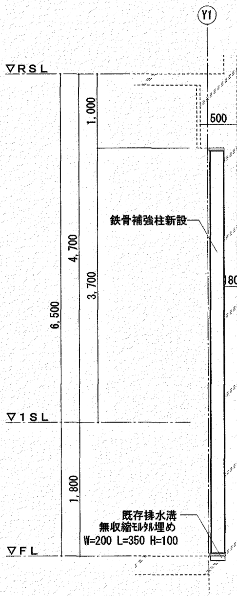
TC1部 断面詳細図(改修後) S=1/50
