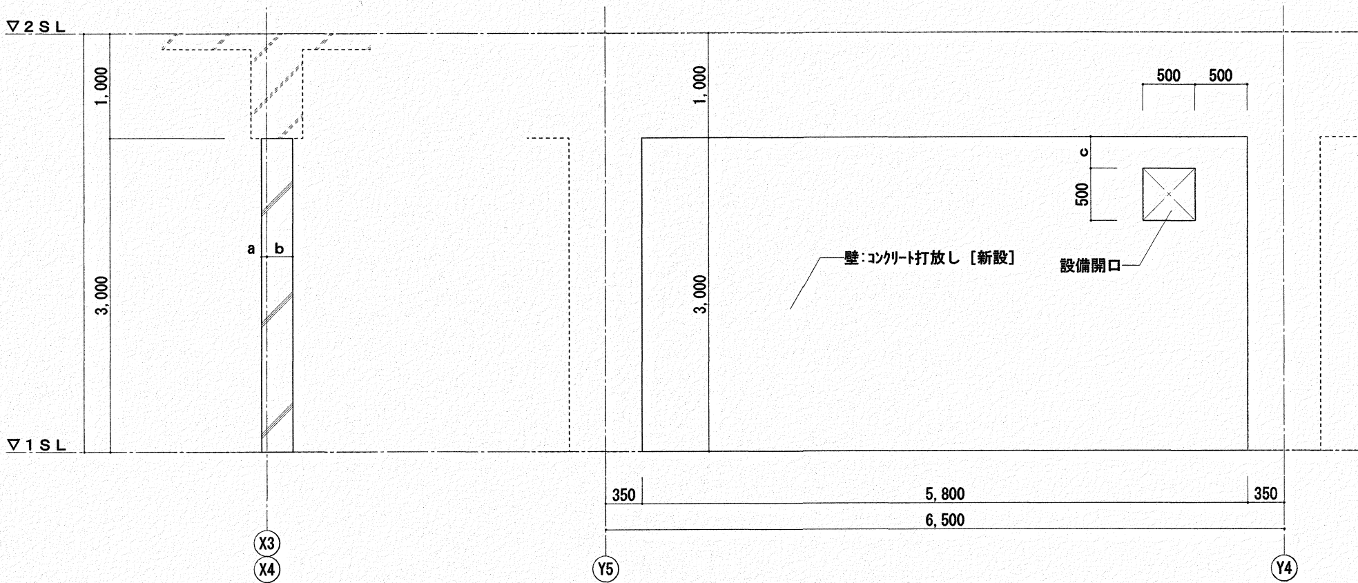
NW30A・B部 断面詳細図 S=1/50
