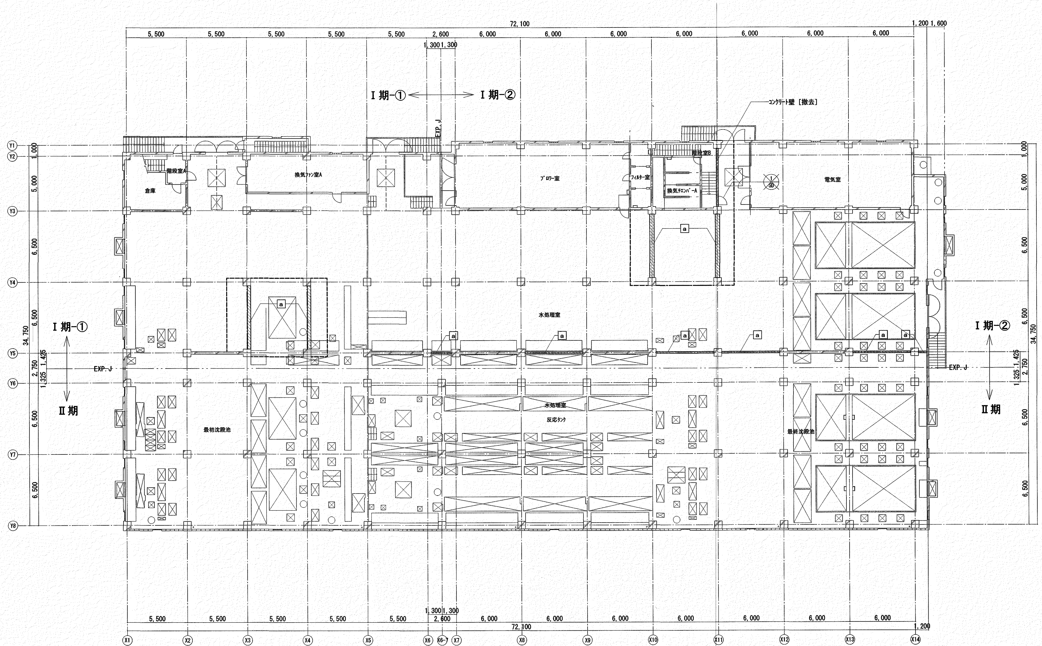
〔水処理棟〕1階平面図(改修前) S=1/200
