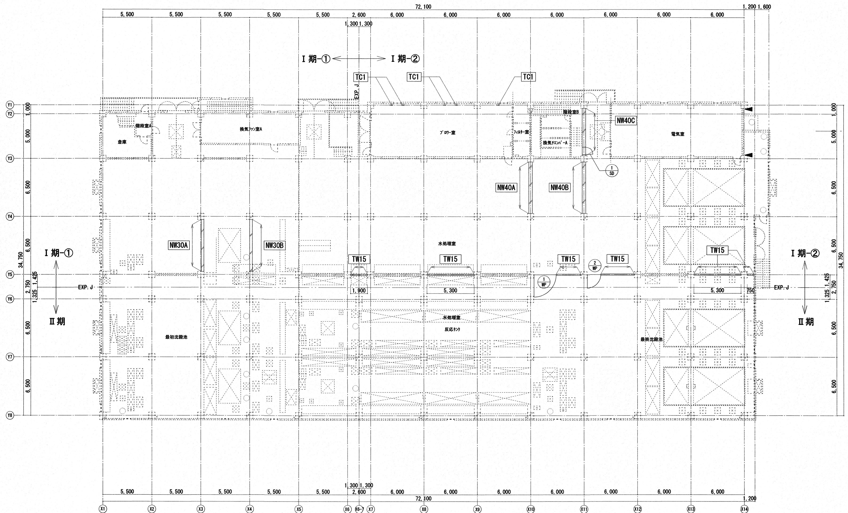
【水処理棟】1階平面図(改修後) S=1/200
