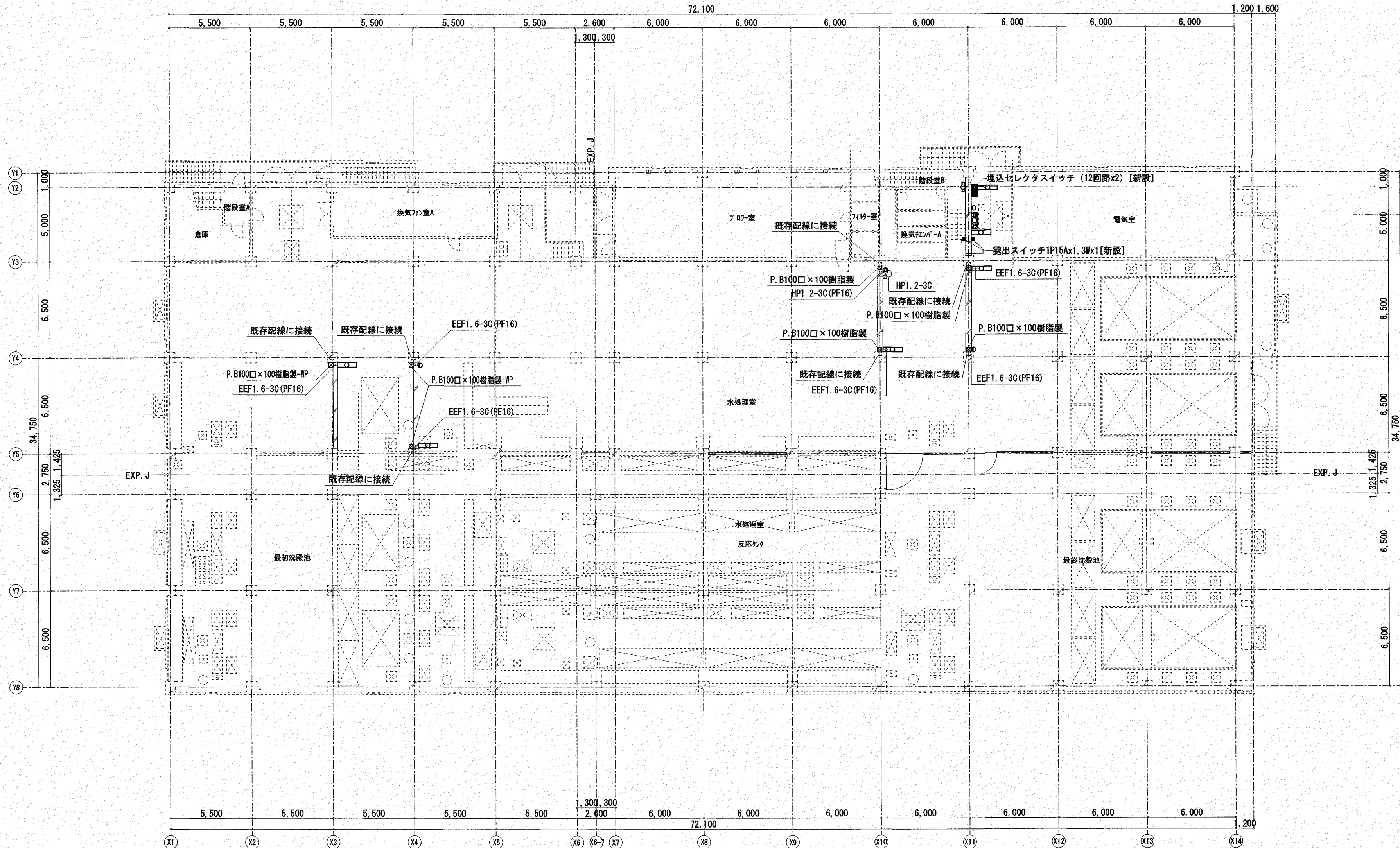
[水処理棟] 1階電気設備平面図(改修後) S=1:200 ※施工前に既存設備の調査を行うこと
