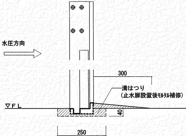
止水扉参考断面詳細図 S=1/10
