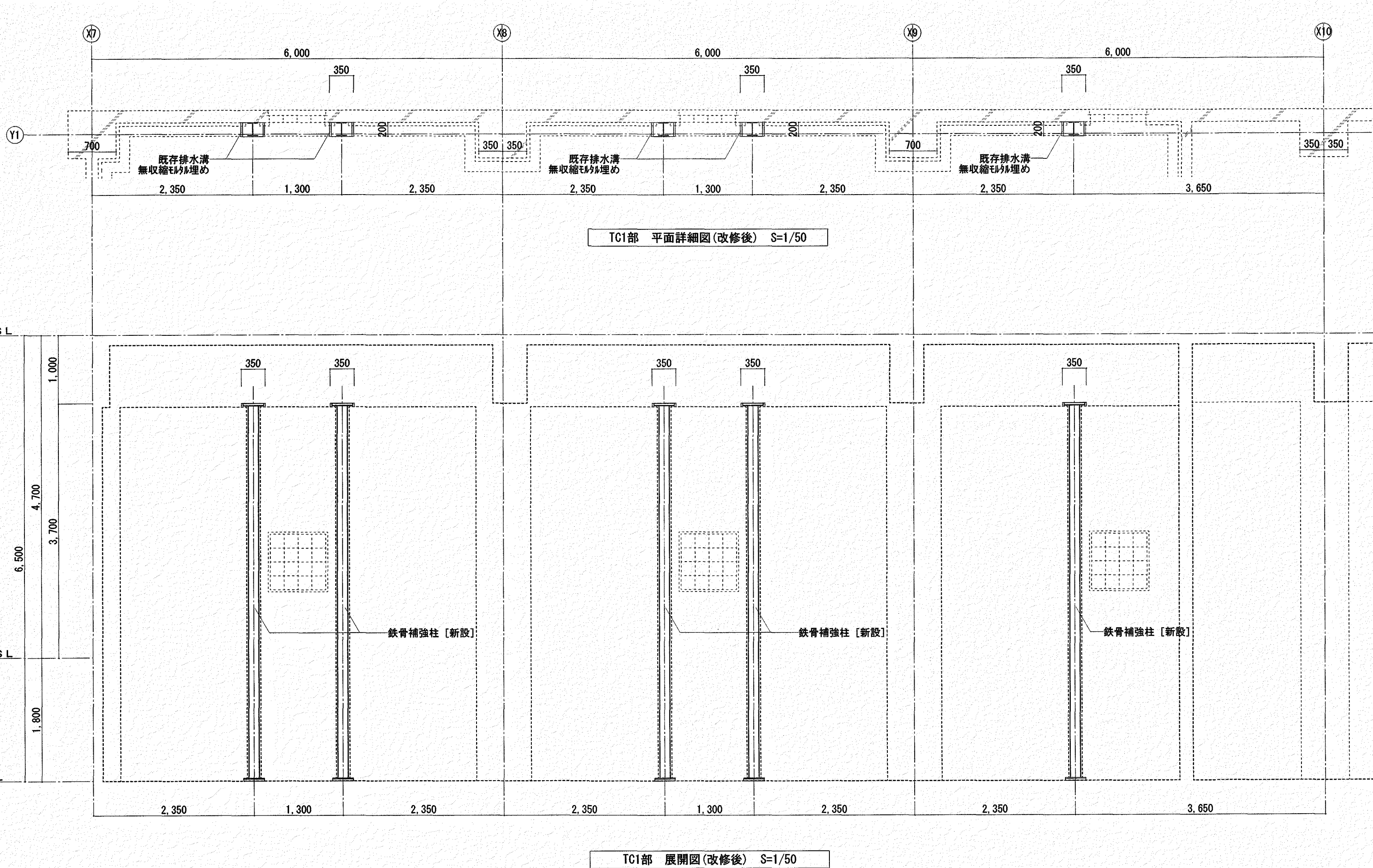
TC1部 展開図(改修後) S=1/50
