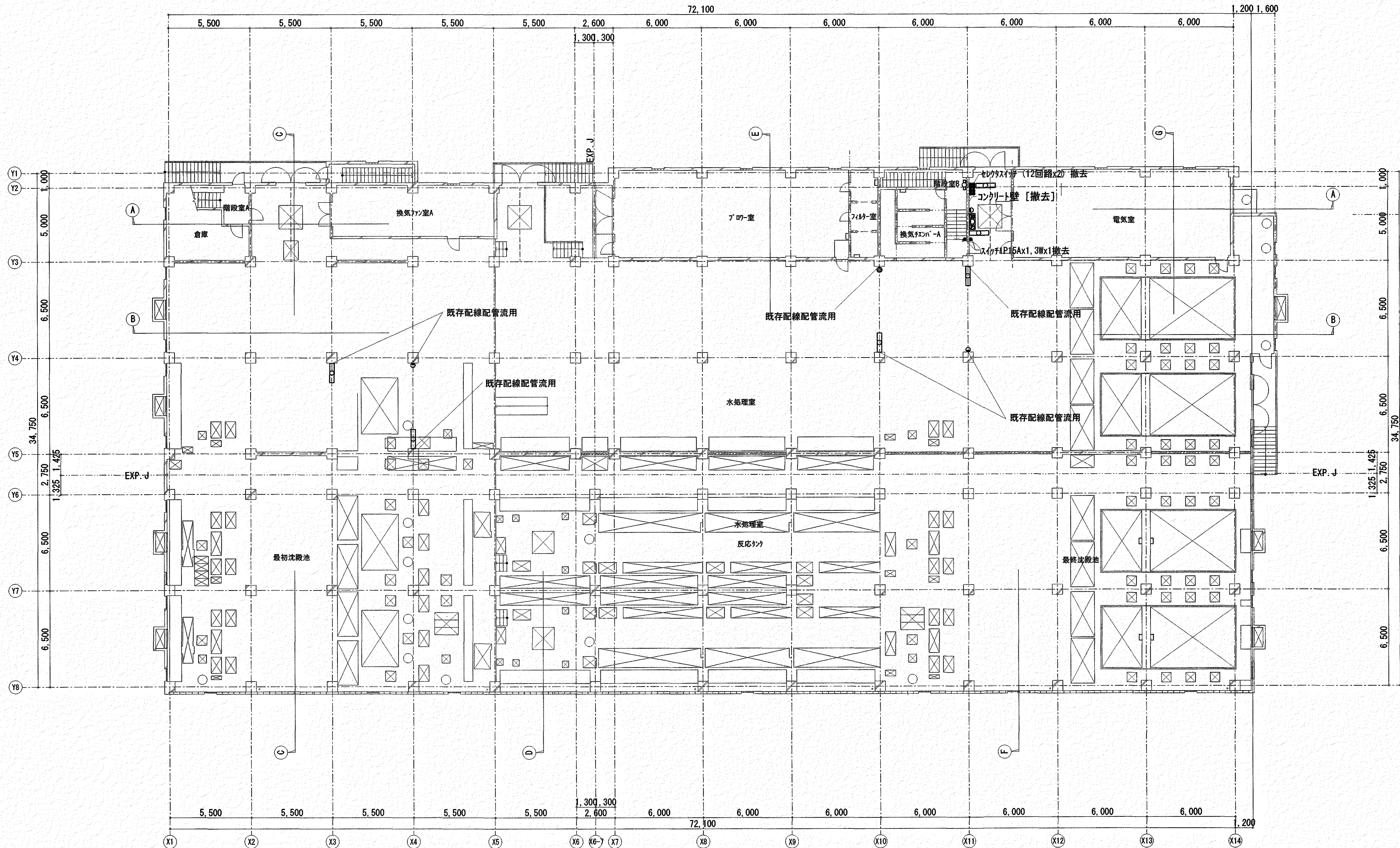
[水処理棟] 1階電気設備平面図(改修前) S=1:200
