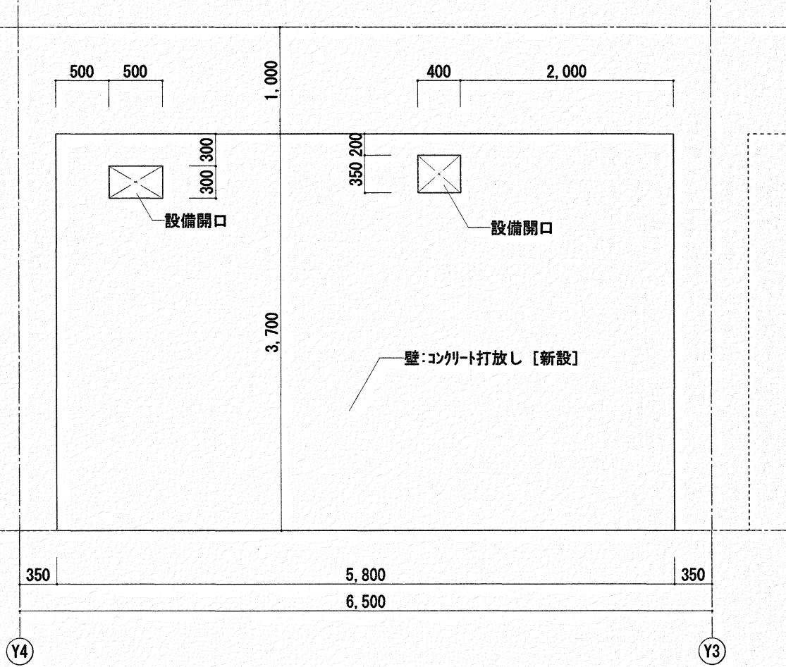
NW40B部 X11通り展開図 S=1/50
