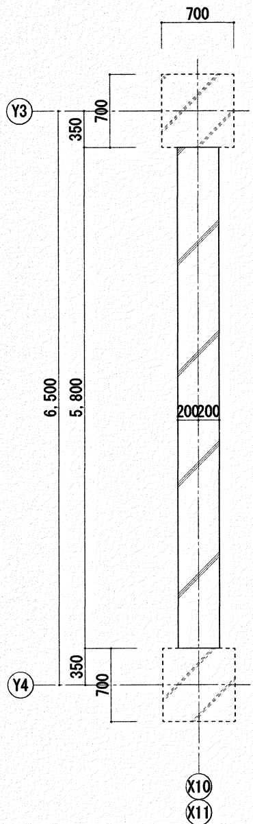
NW40A・B部 平面詳細図 S=1/50
