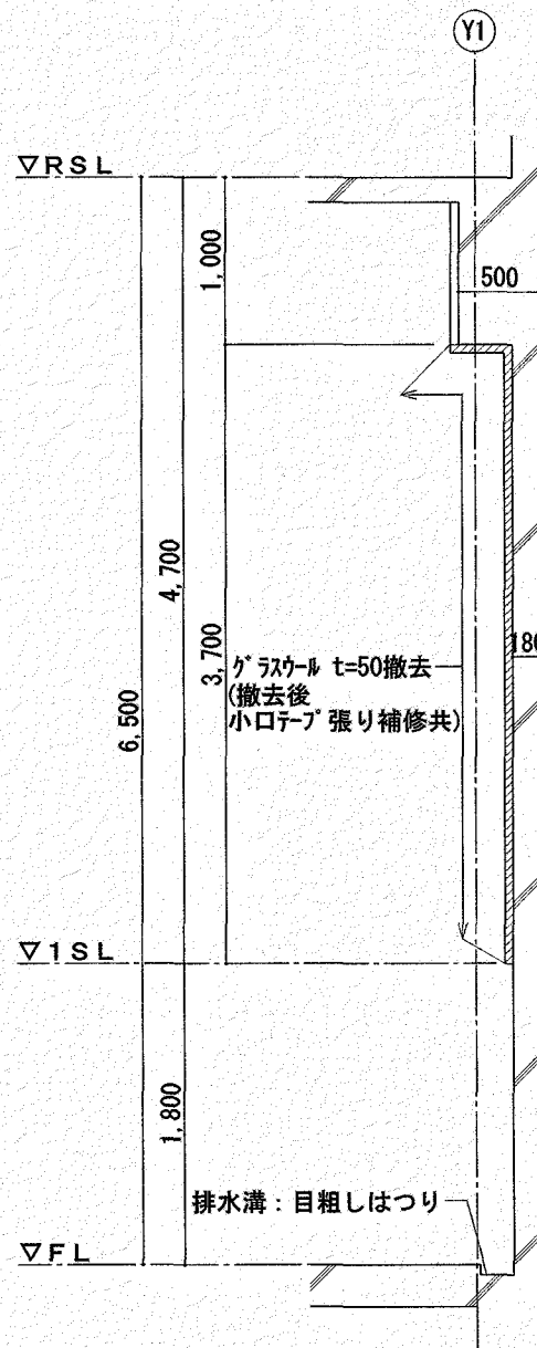
TC1部 断面詳細図(改修前) S=1/50
