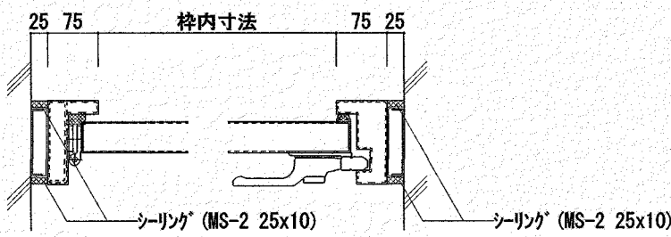
止水扉参考平面詳細図 S=1/10
