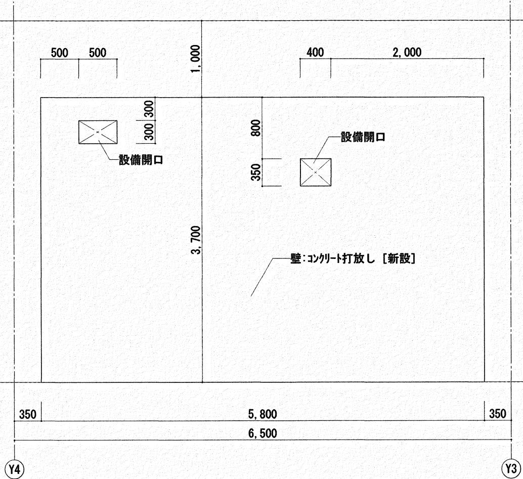
NW40A部 X10通り展開図 S=1/50
