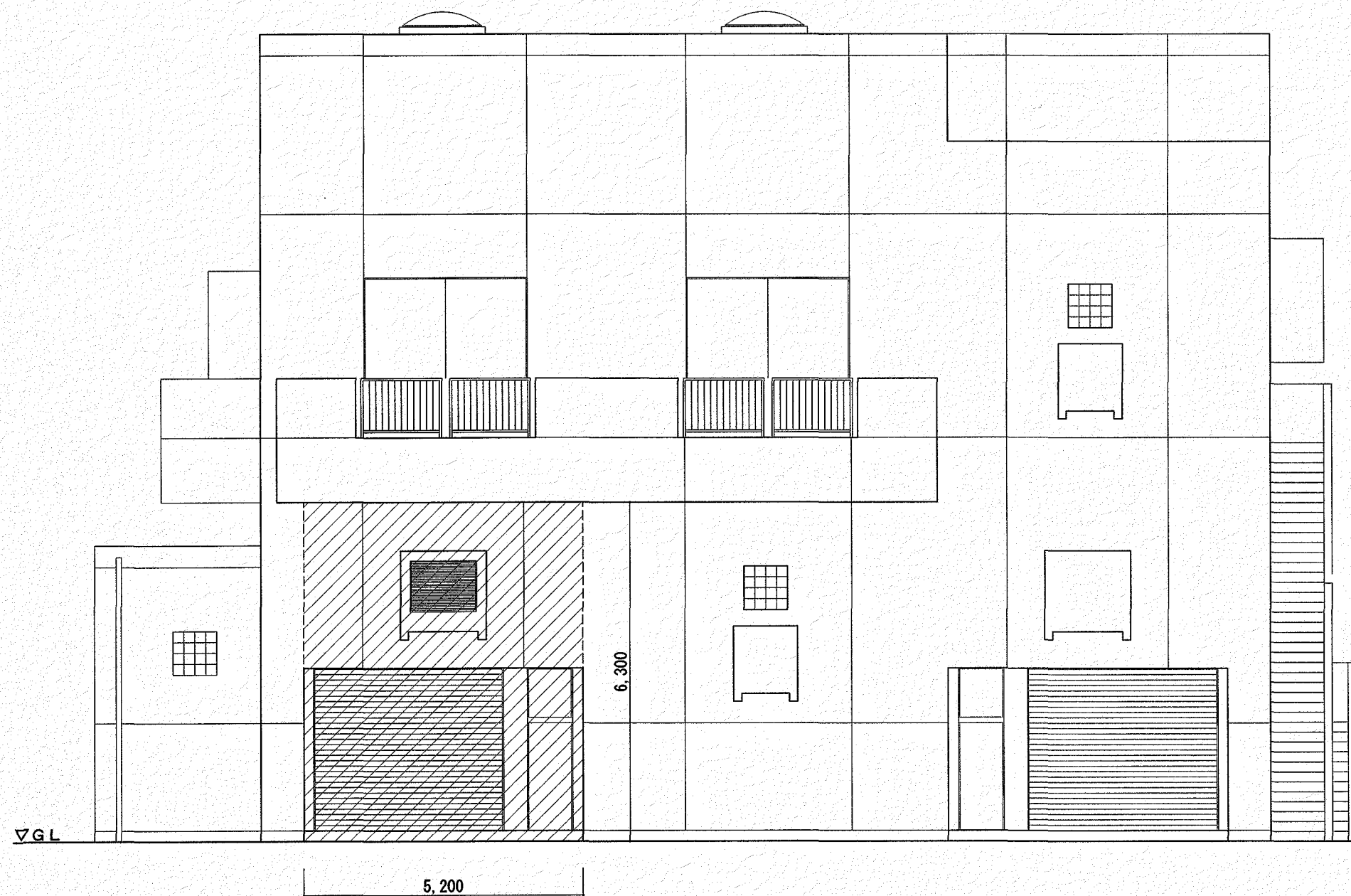
南立面図(改修前) S=1/100
