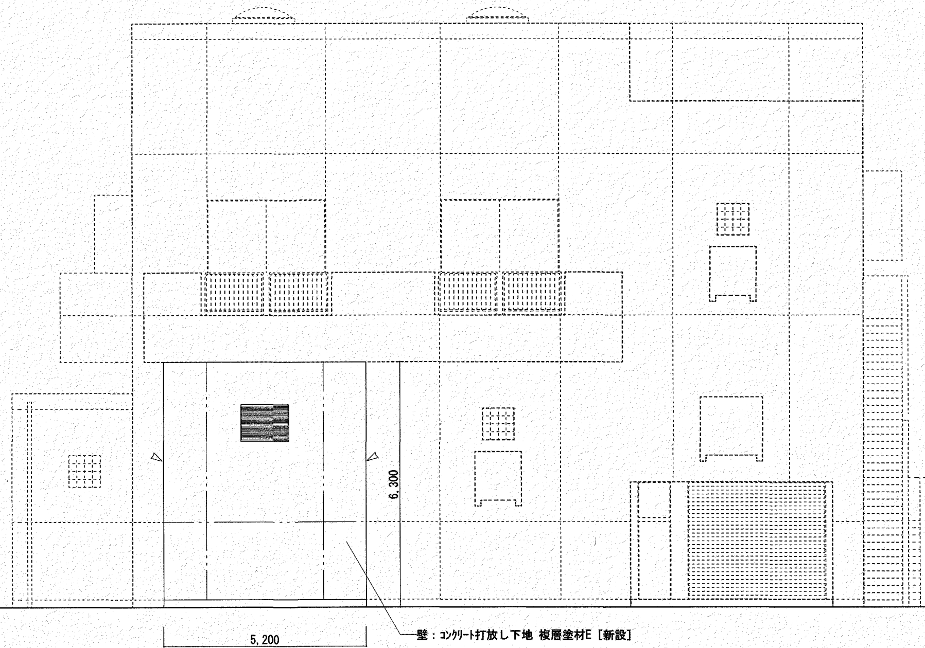
南立面図(改修後) S=1/100
