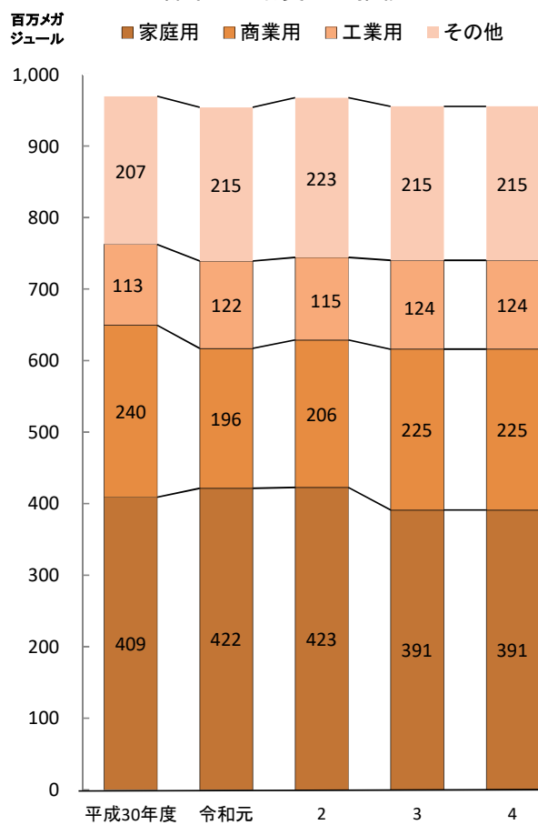
都市ガス消費量の推移
