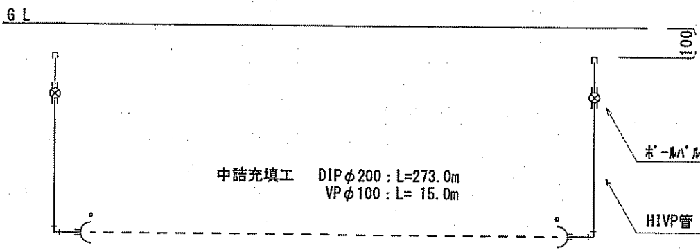
廃止管中詰充填図 S=1:Free
