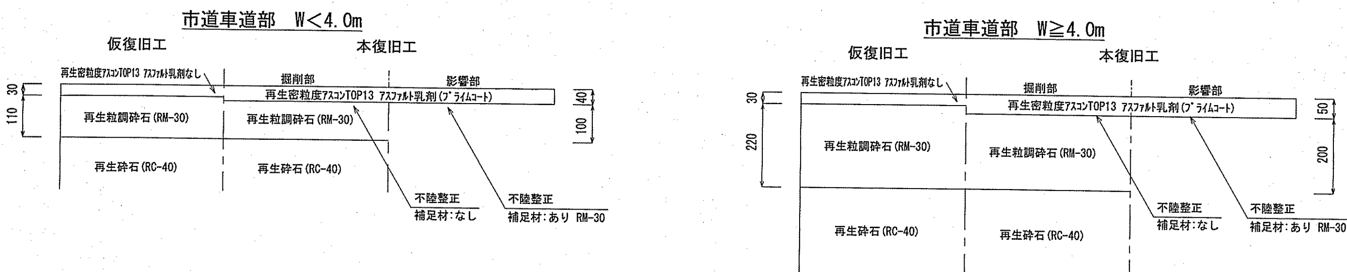
舗装構成図 S=Free
