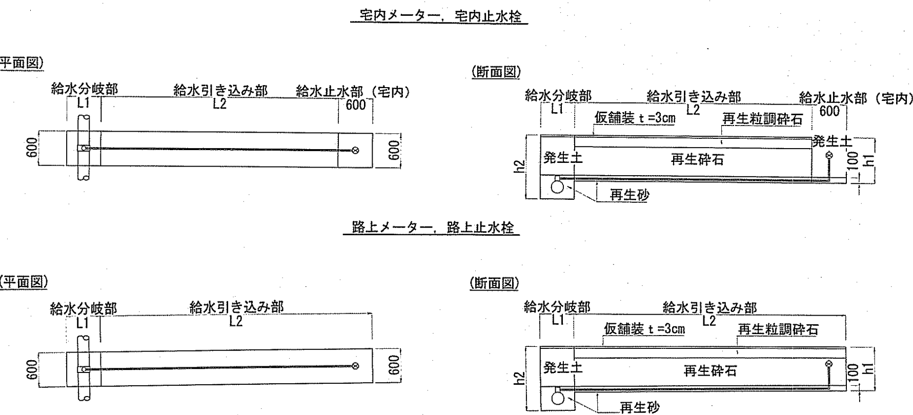
切替標準断面図 S=1:Free
