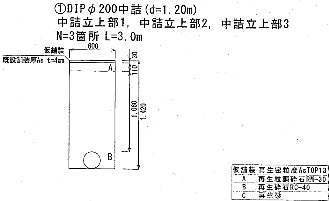
廃止管土工図 S=1:30
