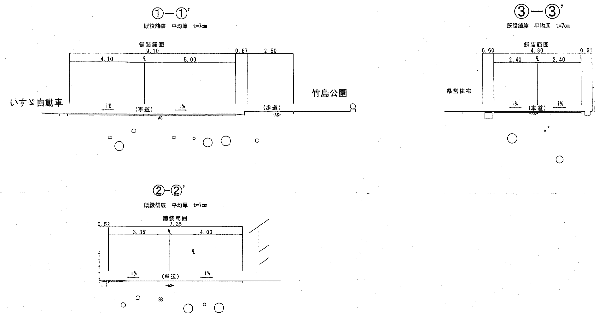
横断図 S=1:50
