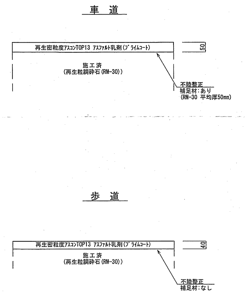
舗装構成図 S=1:10
