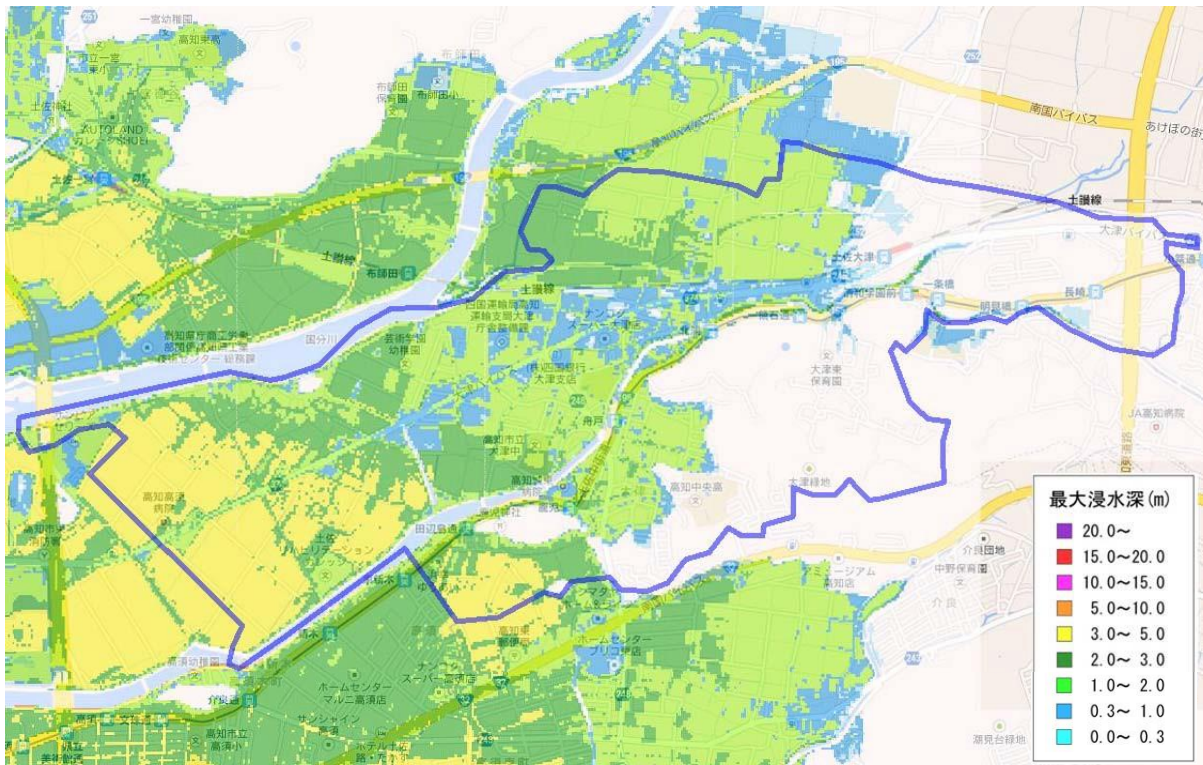
図 3-8 大津小学校区の津波浸水予測図
