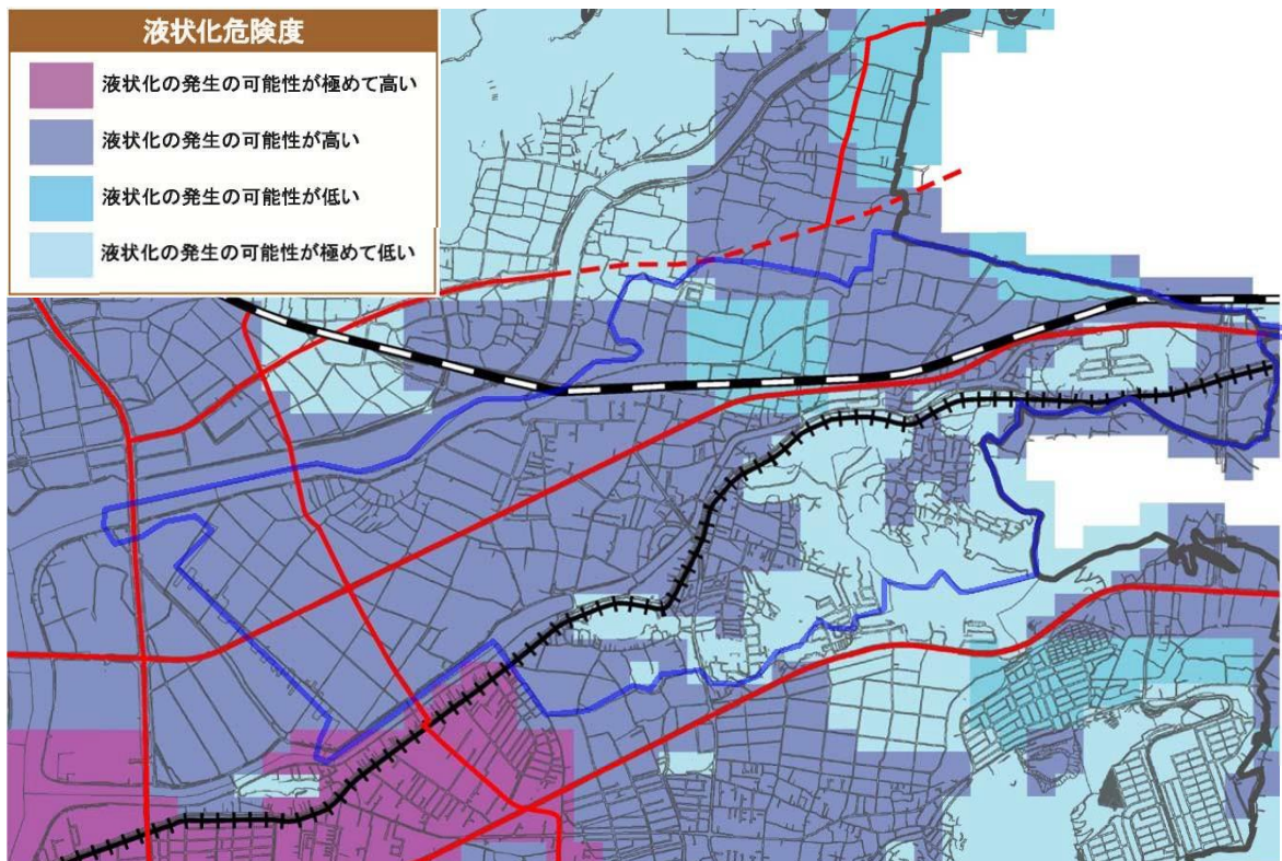
図 3-7 大津小学校区の液状化危険度図
