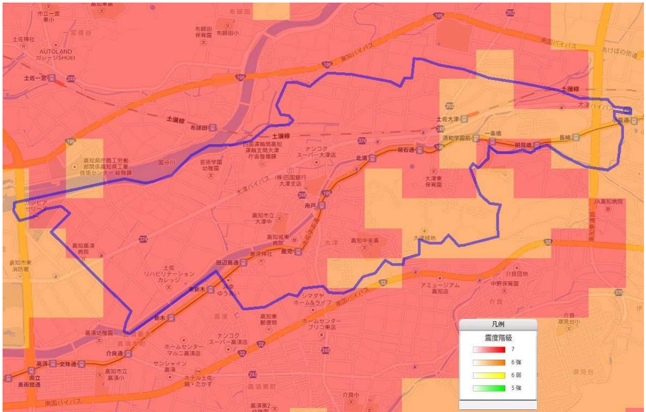
図 3-6 大津小学校区の震度分布図
