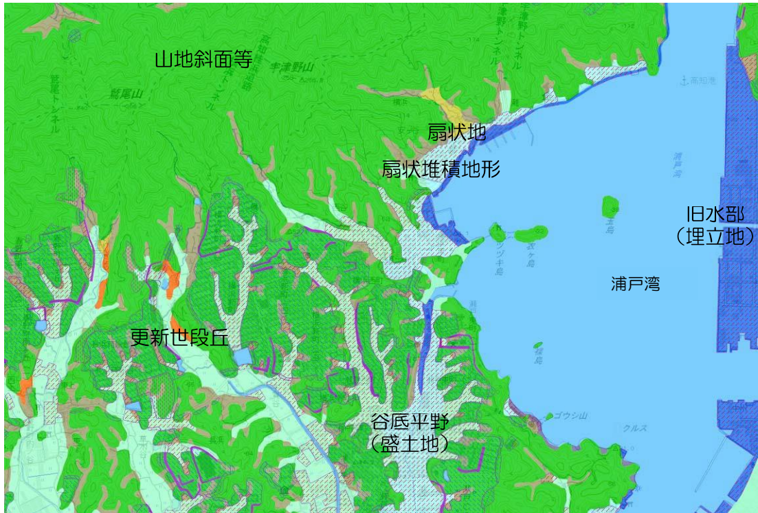
図4-2 横浜小学校区周辺の地形の成り立ち
