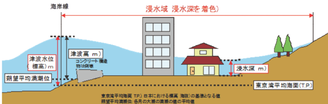
図2 津波高及び津波浸水深のイメージ
