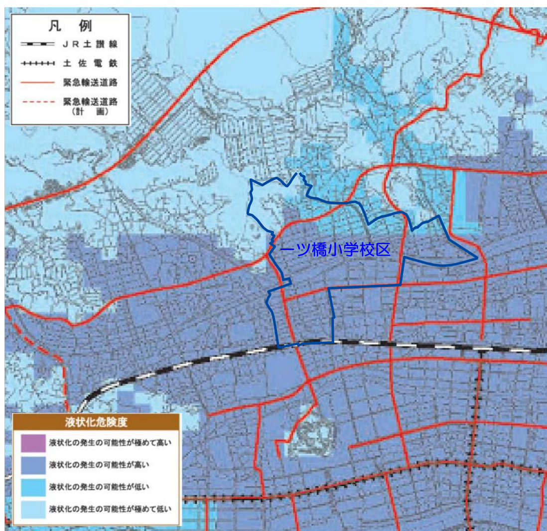
図 3-7 一ツ橋小学校区における液状化危険度図
