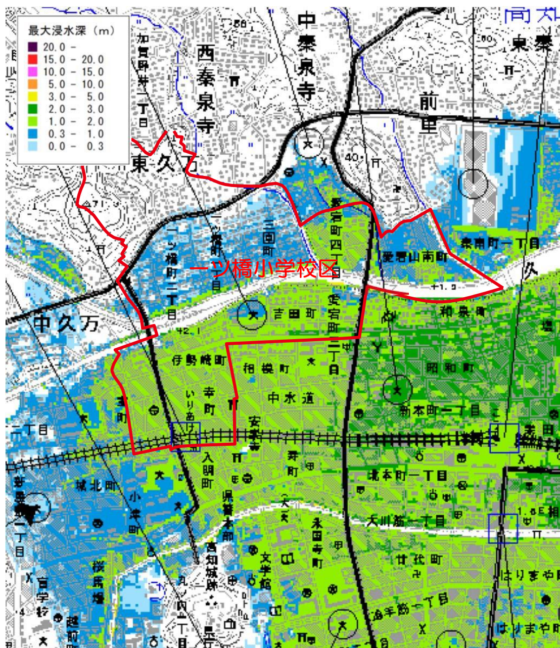
図3-9 一ツ橋小学校区における津波浸水予測図
