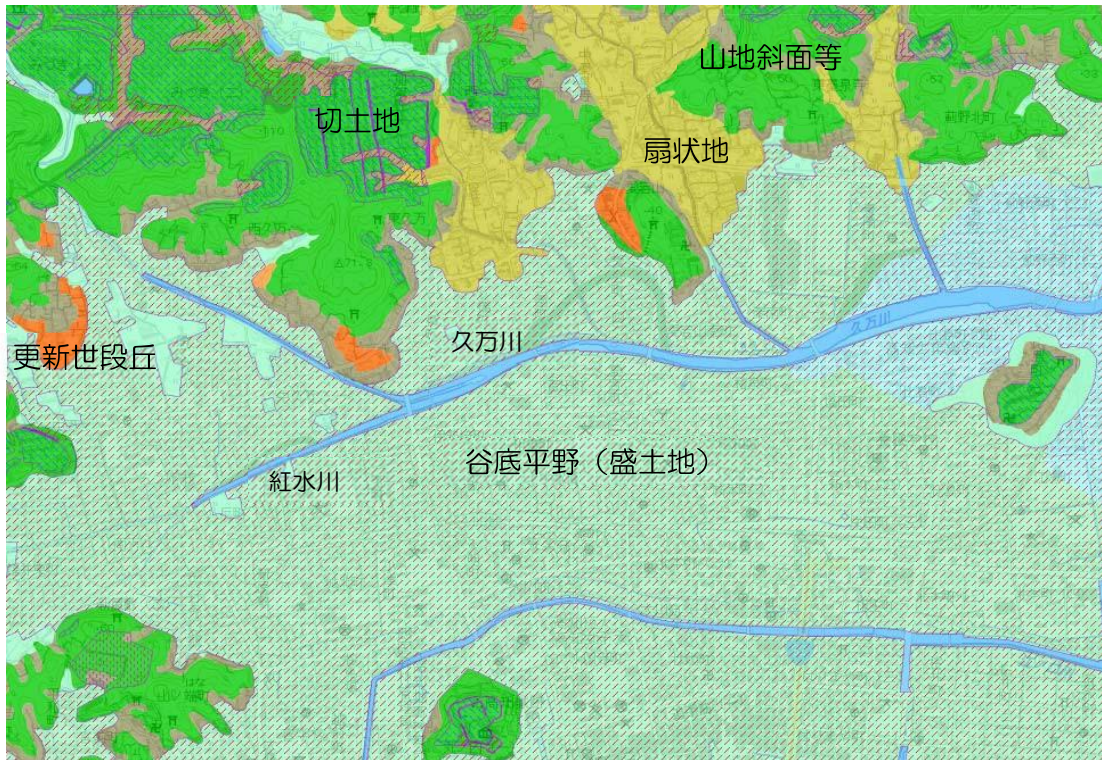
図4-2 一ツ橋小学校区周辺の地形の成り立ち
