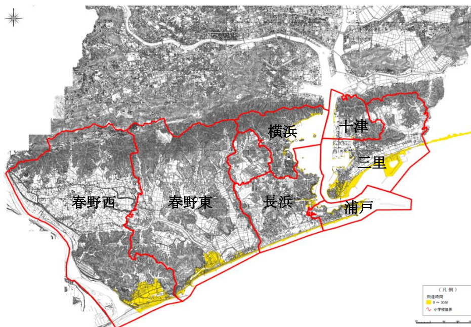
図3 高知市の事前避難対象地域(黄色箇所)
