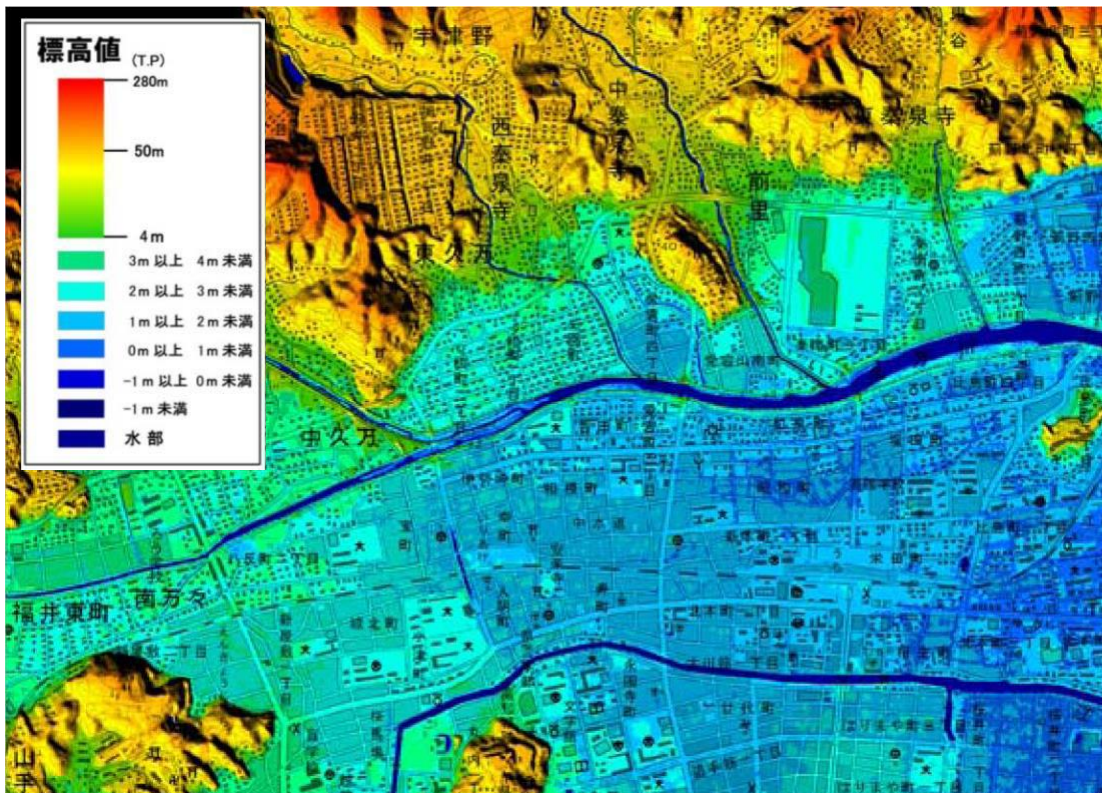
図4-3 一ツ橋小学校区周辺の標高値
