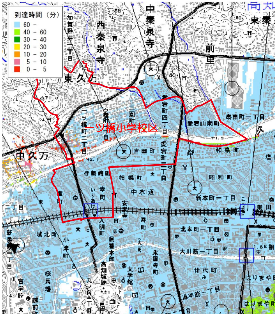
図 3-8 一ツ橋小学校区における津波浸水予測時間図（浸水深 30cm）
