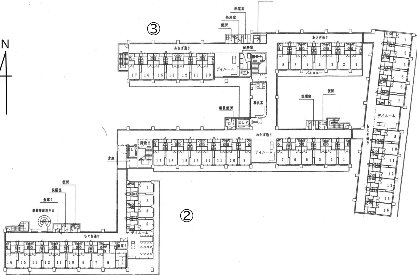
敷地2段目3階平面図
