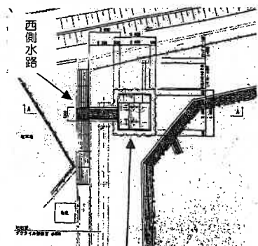
体育館北ポンプ場(本宮町排水機場)
