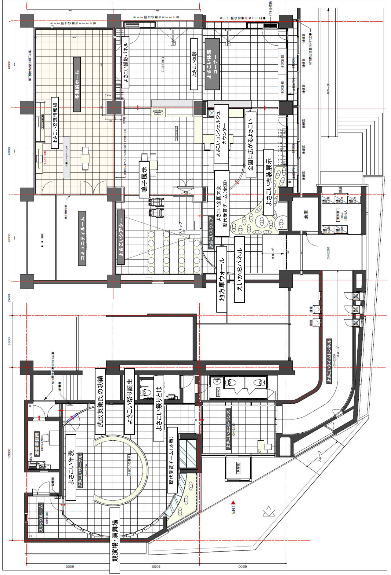
高知よさこい情報交流館 平面図
