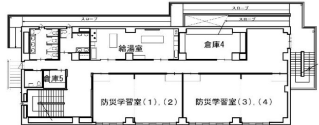
2階平面図
