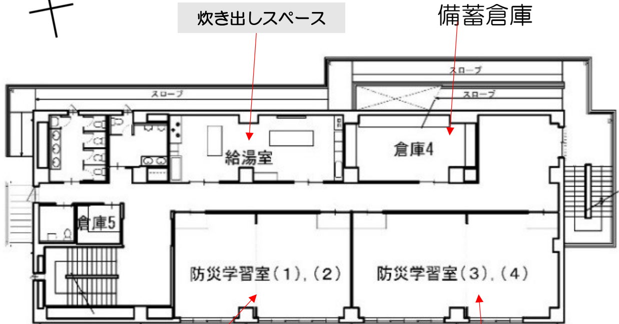
2階平面図
