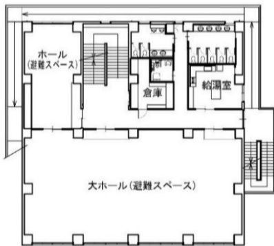
3階平面図
