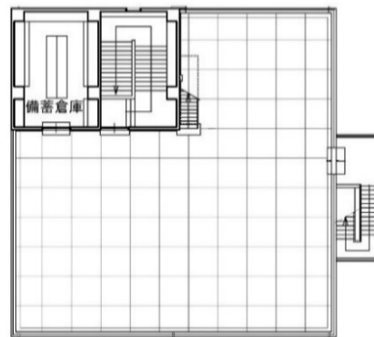
屋上平面図
