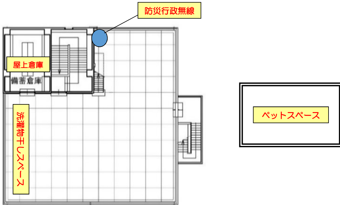
屋上平面図
