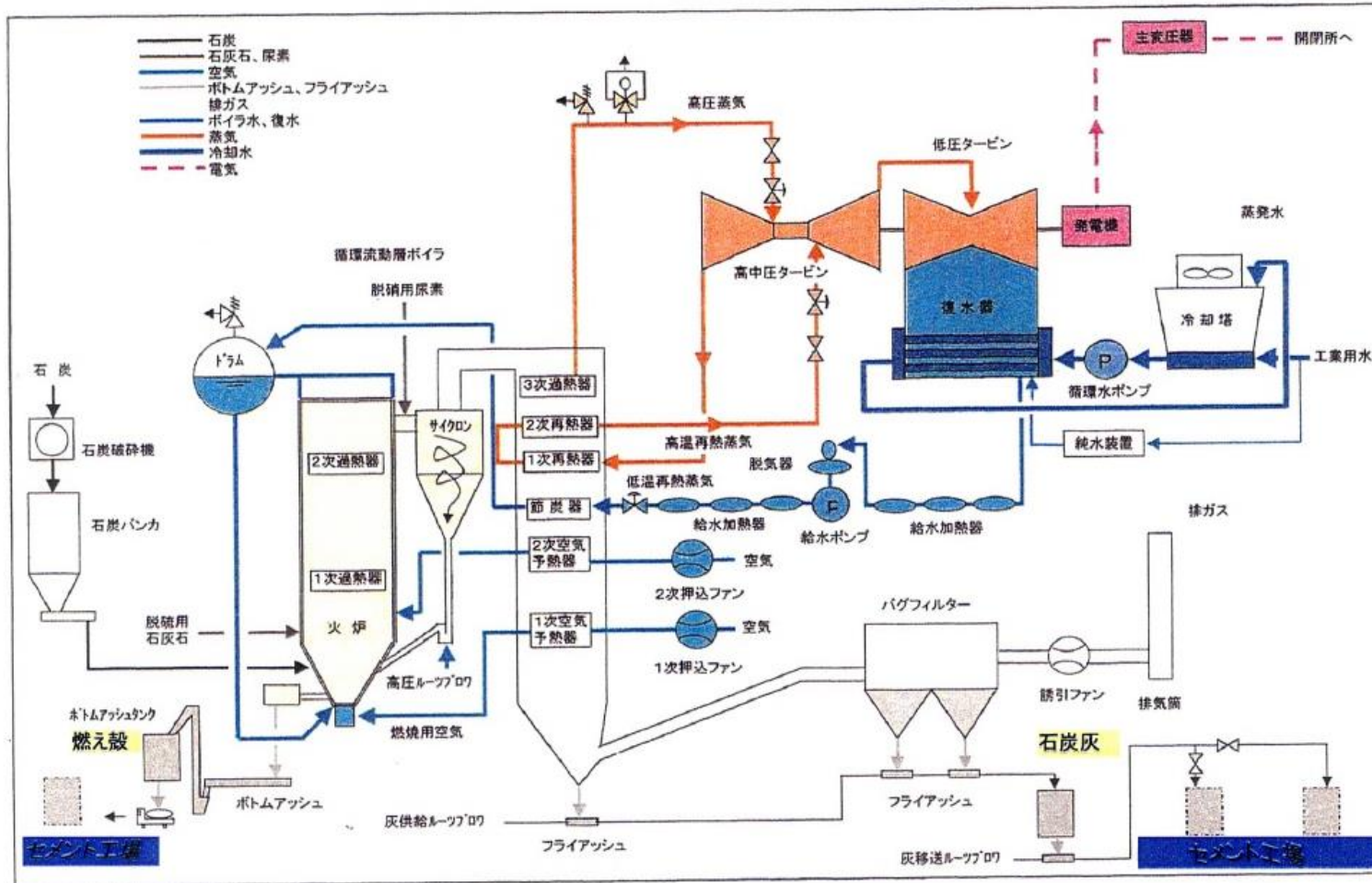
図-1 発電所フロー図
