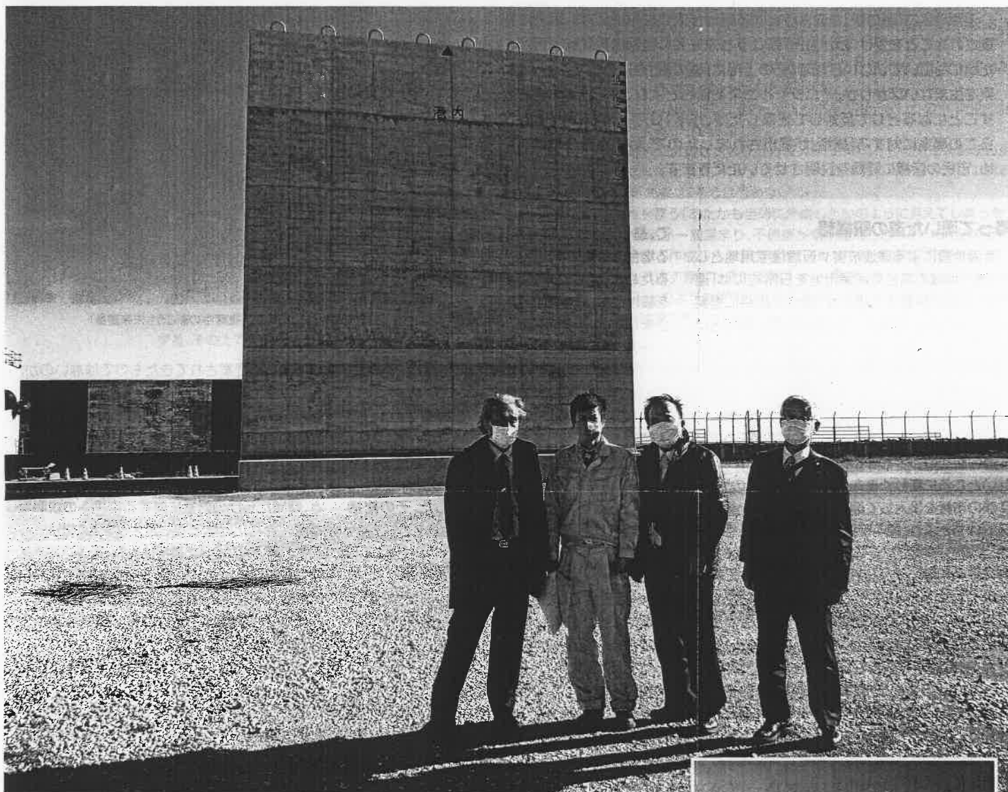
高知新港前で津波をやわらげるために沈める大型ケーソン。国土交通省の若手職員から現地での説明を受けました。
