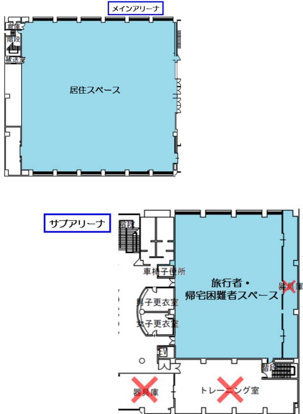
配置計画図（3階）
