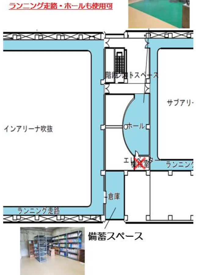
配置計画図（4階）
