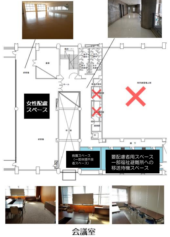
配置計画図（2階）
