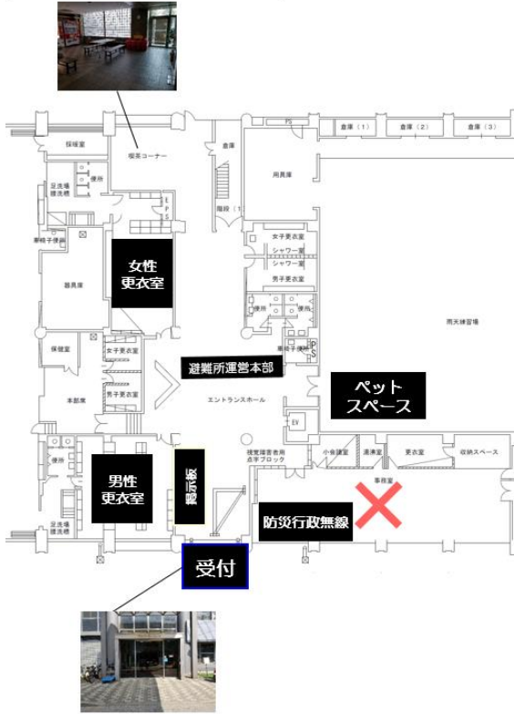
配置計画図（3階）
