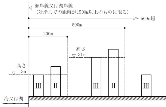
図.1 地表面粗度区分
