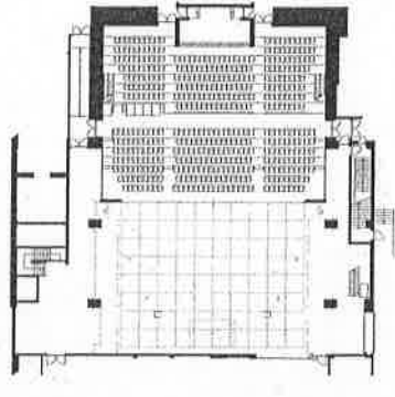
1階平面図 | First floor plan
