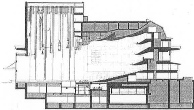
長手方向断面図 | Longitudinal section
