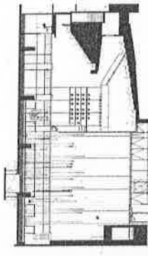
観客方向断面図 | Longitudinal section
