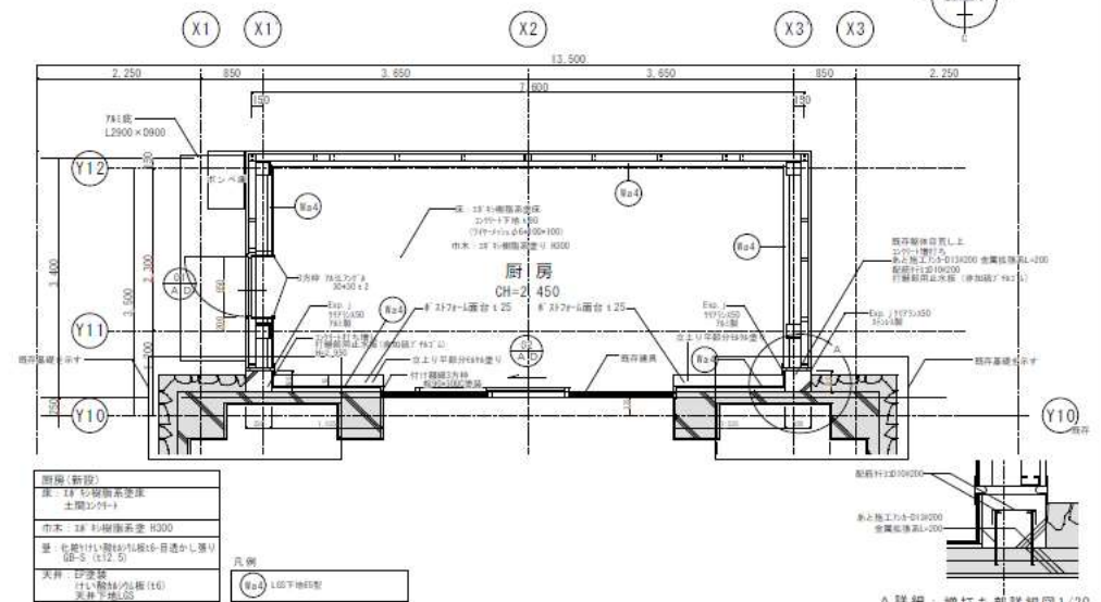
A 詳細: 増打ち部詳細図 1/20
