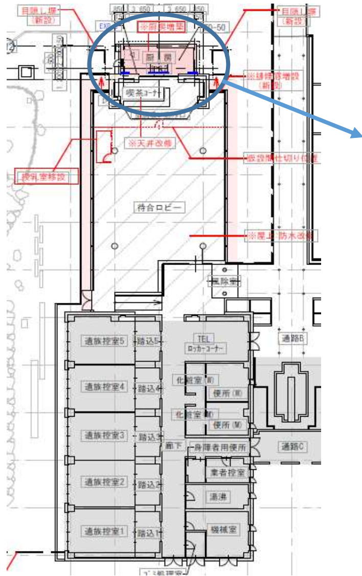
改修平面詳細図 1/50
