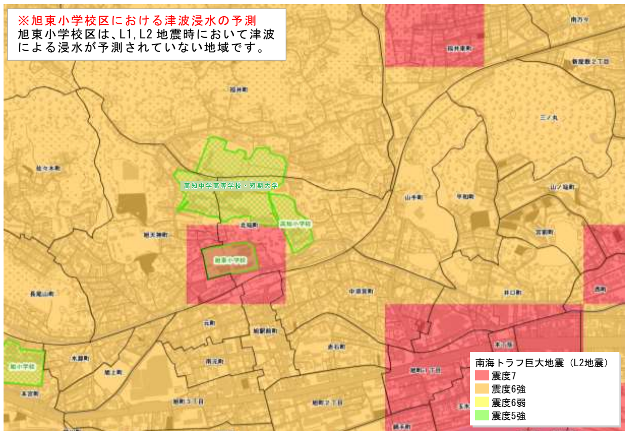
図 3-2 南海トラフ地震（L2地震）が発生した場合の震度分布
