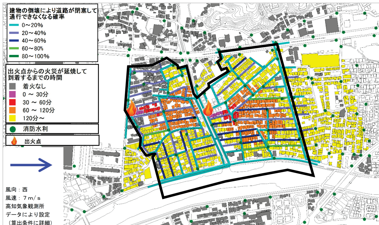
図 3-9 火災の延焼・道路の閉塞についてのシミュレーション結果
