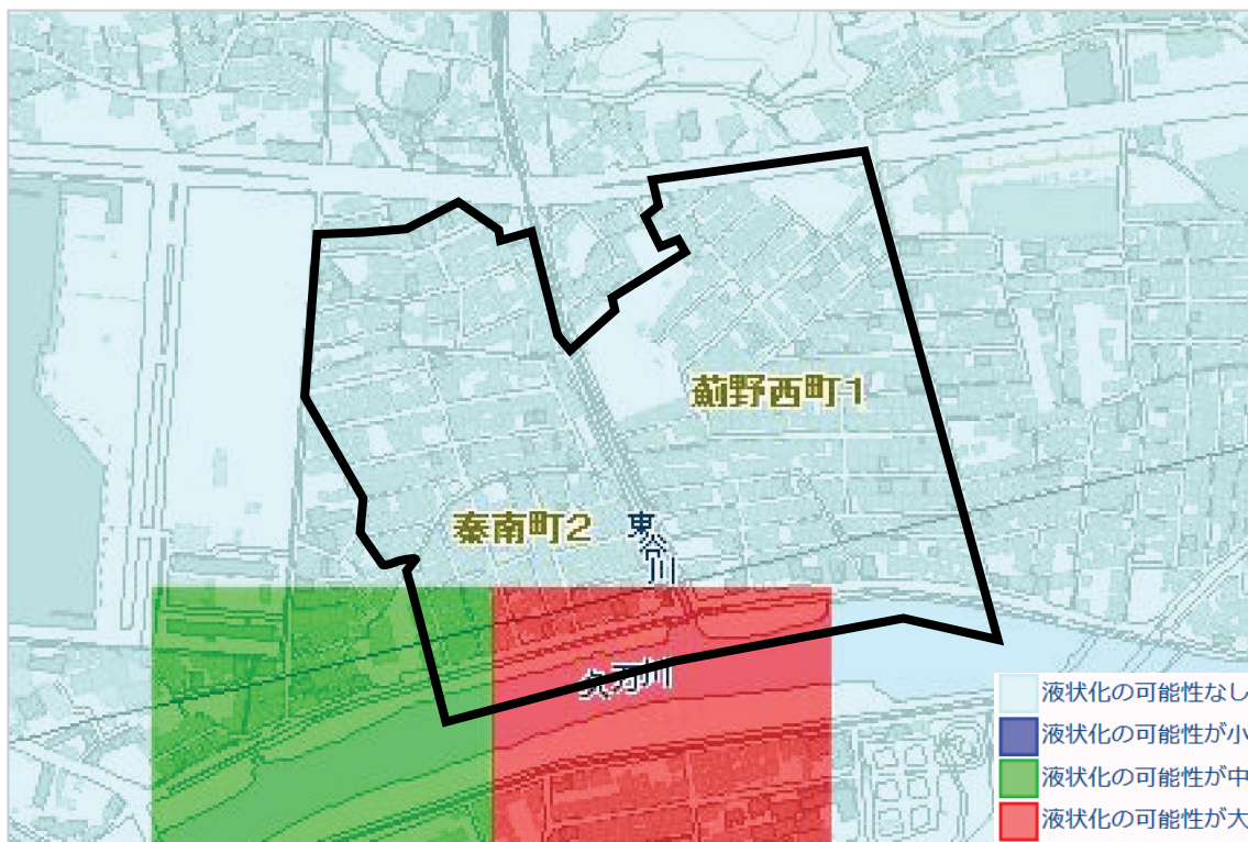
図 3-6 L2地震 薊野西町1丁目、秦南町2丁目の液状化の可能性
