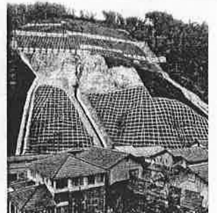
完成した鏡的洲の山腹崩壊の修復工事
