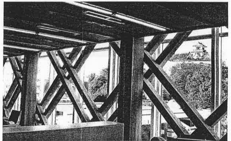
高知県自治会館は木材の多様な活用と新技術が活かされています
